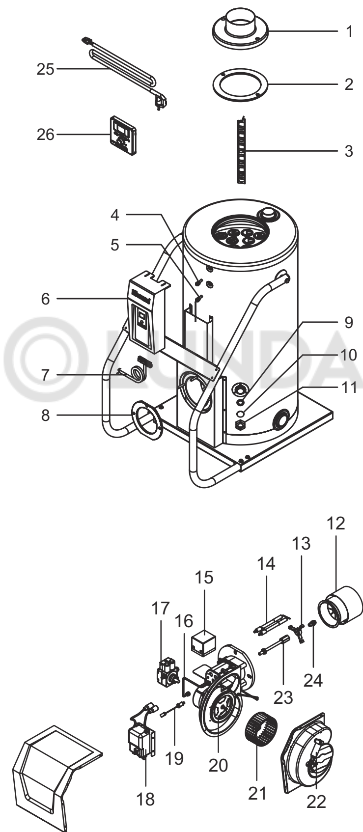
Рисунок 12. Каталог запчастей KSO 58/81.
