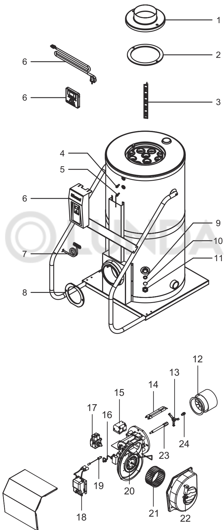
Рисунок 13. Каталог запчастей KSO 116/174.
