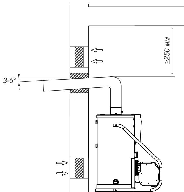
Рисунок 7. Система дымоудаления.
