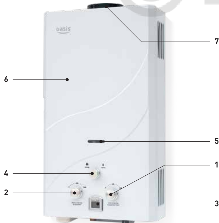
Рис. 1. Аппарат водонагревательный проточный газовый бытовой «OASIS» 1 - ручка водяного регулятора; 2 - ручка газового регулятора; 3 - цифровой индикатор температуры горячей воды; 4 - переключатель зима/лето; 5 - окно смотровое; 6 - облицовка; 7 - патрубок дымоотвода.
