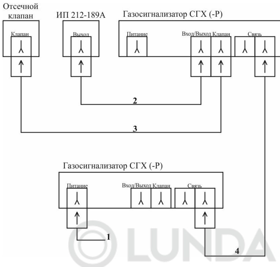
Рис. А2 Пример схемы подключения газосигнализаторов СГХ.
