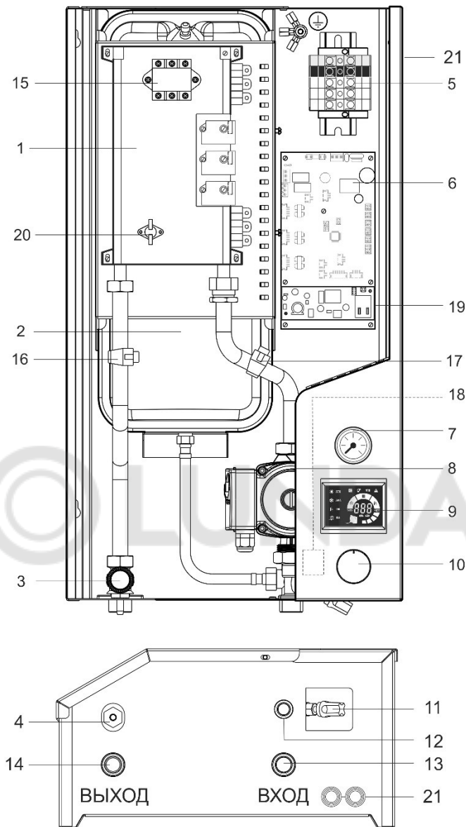
Рисунок 1 - Схема внутреннего устройства электродкотла
