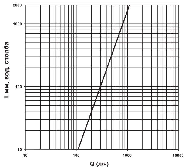
Рис. 5 вентиль «monodet» код 1550
