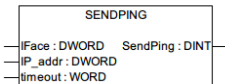
Рисунок 7.16 – Графическое представление функции SENDPING
