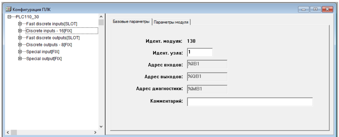
Рисунок 10.2 – Параметры в окне редактора «Конфигурация ПЛК»
