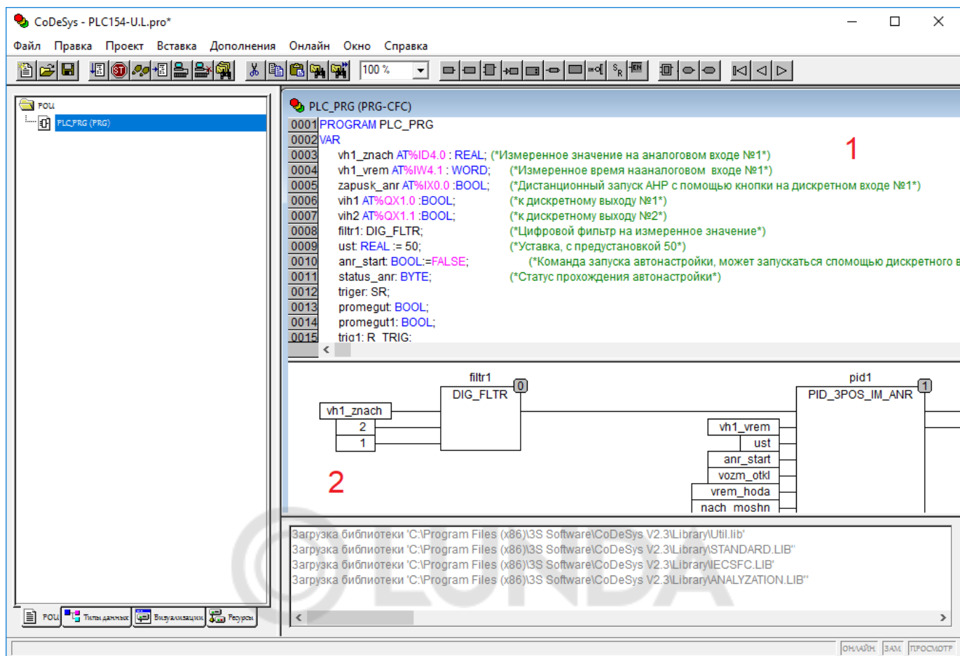
Рисунок 6.15 – Пример окна редактирования: 1 – раздел объявлений; 2 – область кода
