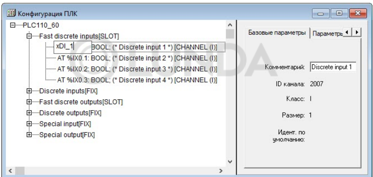
Рисунок 10.9 – Ввод и редактирование имени переменной канала
