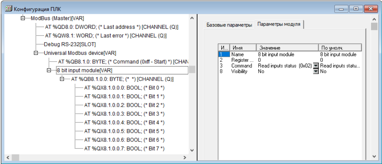
Рисунок 10.26 – Подкаталог канала ввода-вывода
