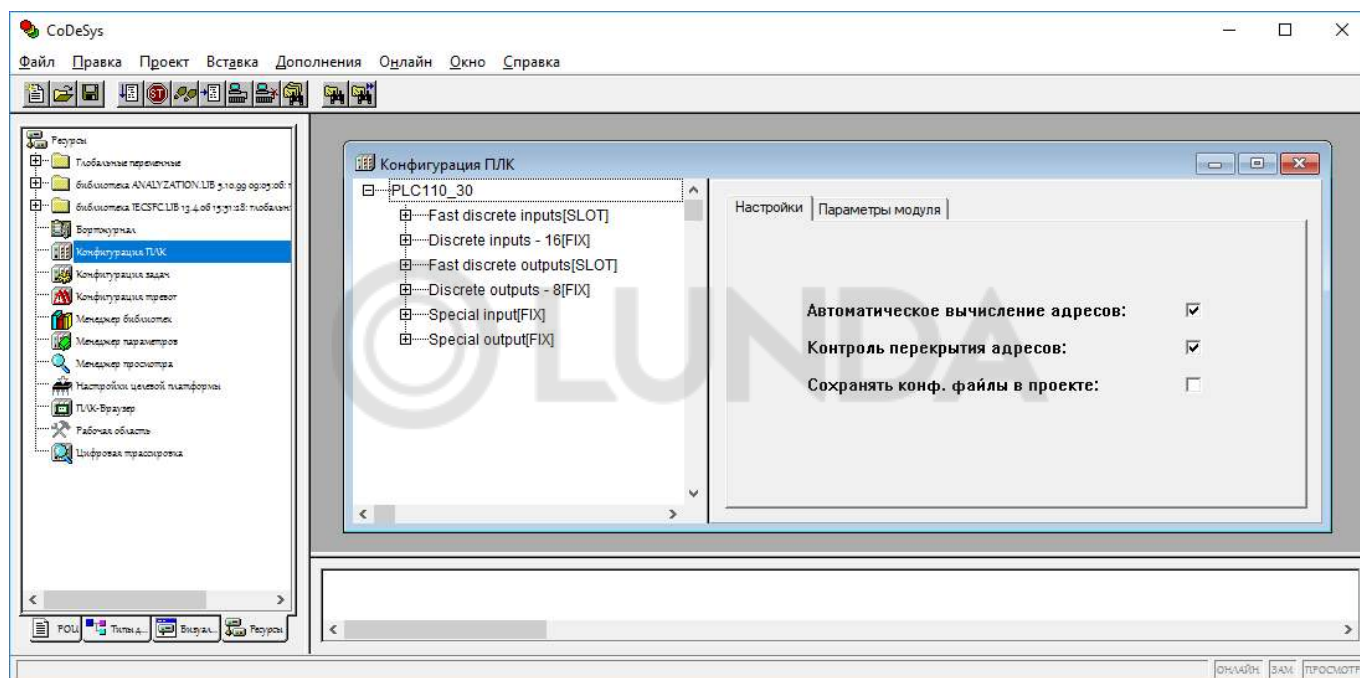
Рисунок 10.1 – Окно редактора «Конфигурация ПЛК»
