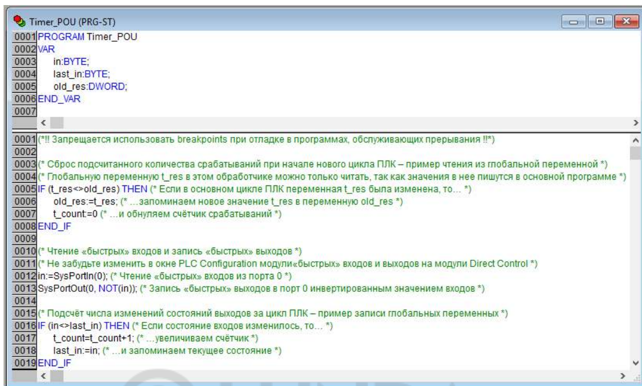
Рисунок 14.5 – Программа обработки высокочастотного таймера («Timer_POU»)
