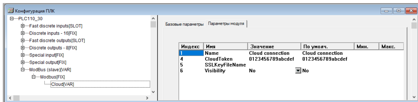
Рисунок 10.59 – Параметры подмодуля Cloud
