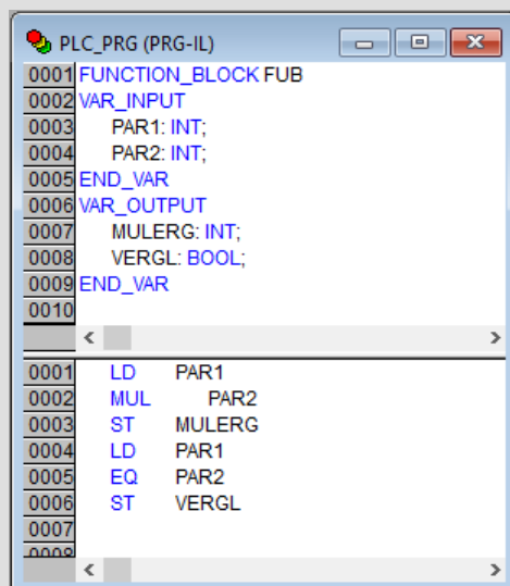
Рисунок 7.3 – Пример записи функционального блока на языке IL
