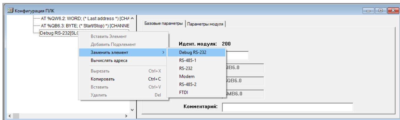
Рисунок 10.36 – Выбор коммуникационных интерфейсов
