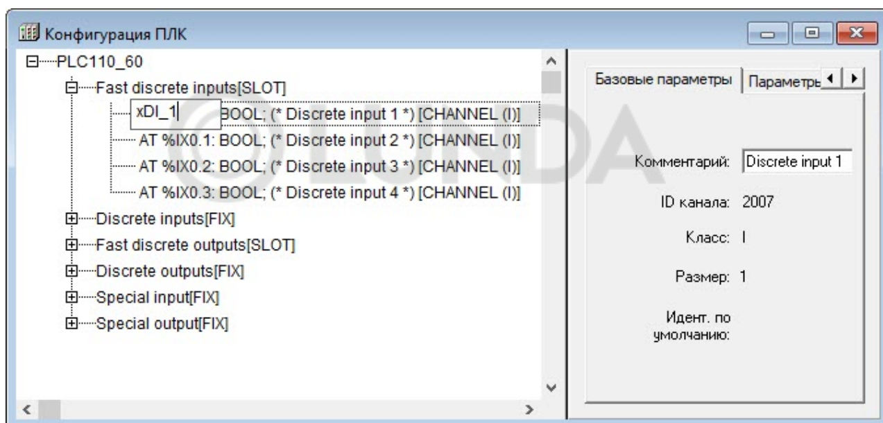
Рисунок 10.9 – Ввод и редактирование имени переменной канала
