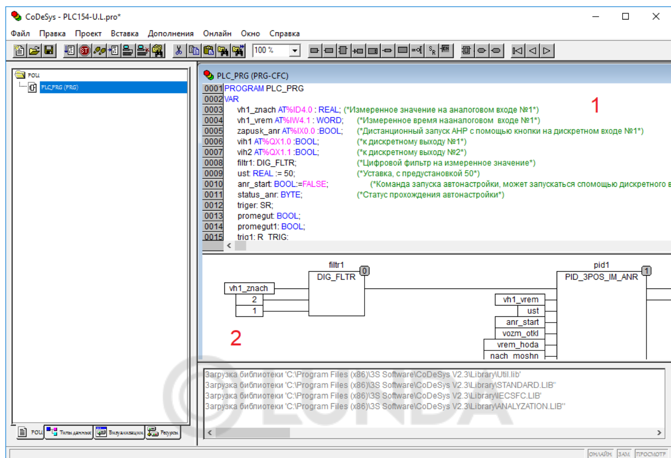
Рисунок 6.15 – Пример окна редактирования: 1 – раздел объявлений; 2 – область кода
