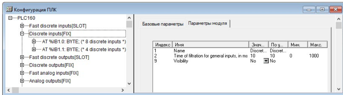
Рисунок 10.16 – Параметры модуля «Дискретные входы» (Discrete input)
