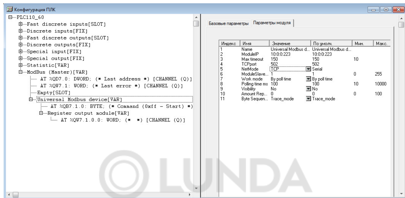
Рисунок 10.60 – Конфигурация модуля при использовании модема
