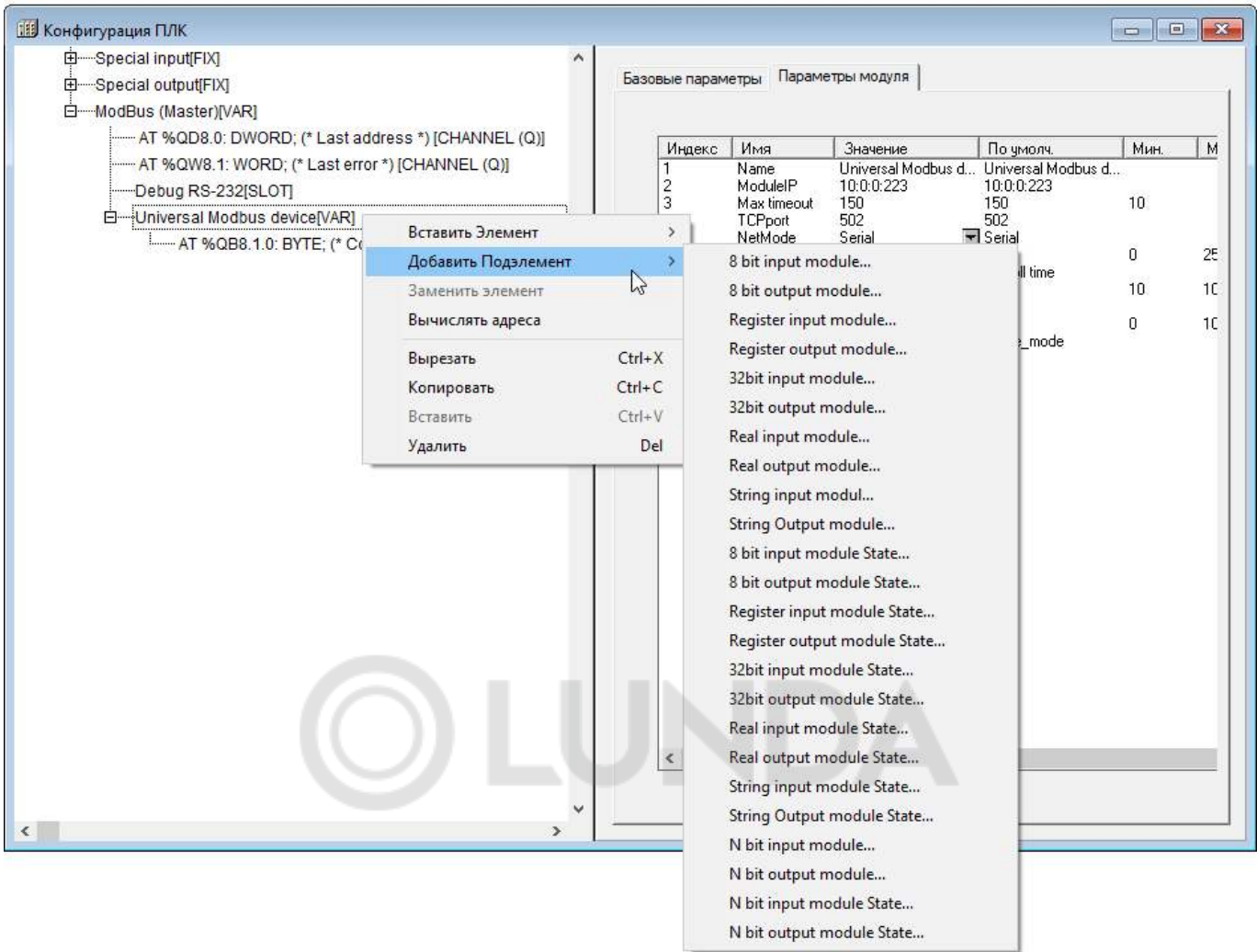
Рисунок 10.25 – Добавление каналов ввода-вывода подмодуля Universal Modbus device
