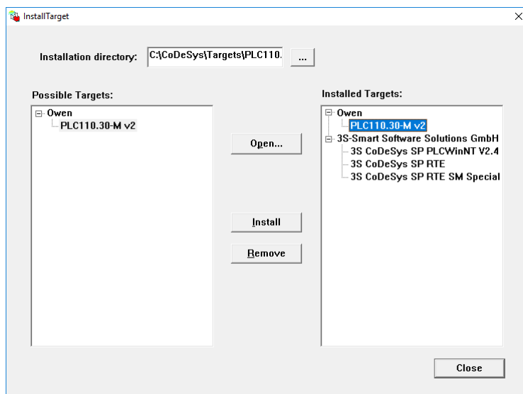
Рисунок 5.2 – Установленный target-файл
