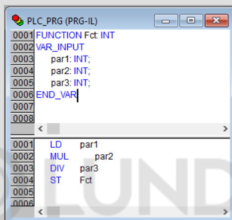
Рисунок 7.2 – Пример записи функции на языке IL
