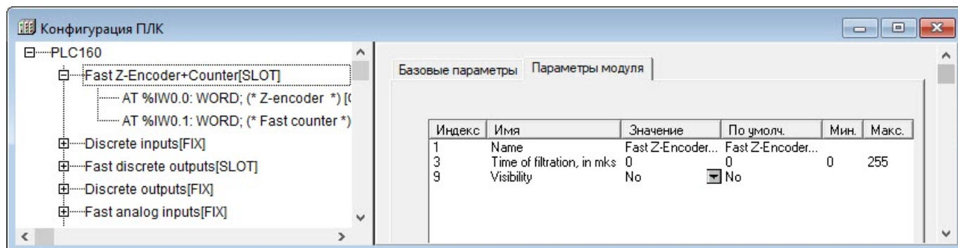
Рисунок 10.15 – Параметры модуля «Высокочастотный Z-энкодер + счетчик»
