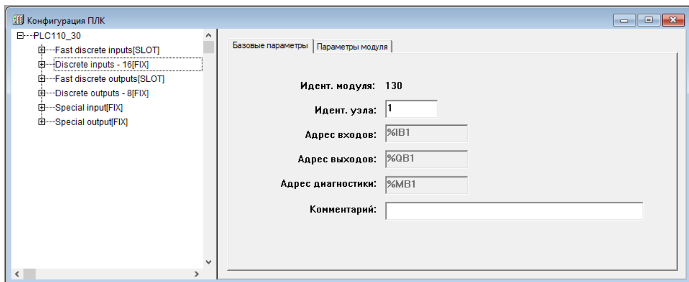
Рисунок 10.2 – Параметры в окне редактора «Конфигурация ПЛК»
