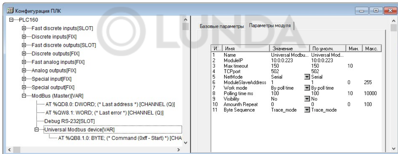
Рисунок 10.24 – Параметры подмодуля Universal ModBus device
