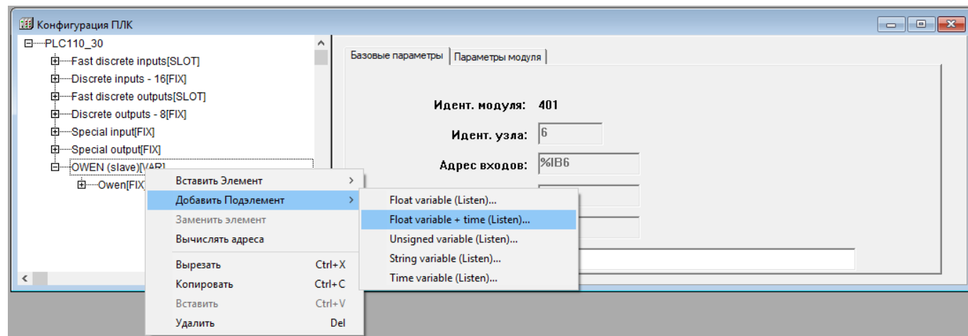
Рисунок 10.42 – Выбор переменных для обмена ПЛК по протоколу OWEN
