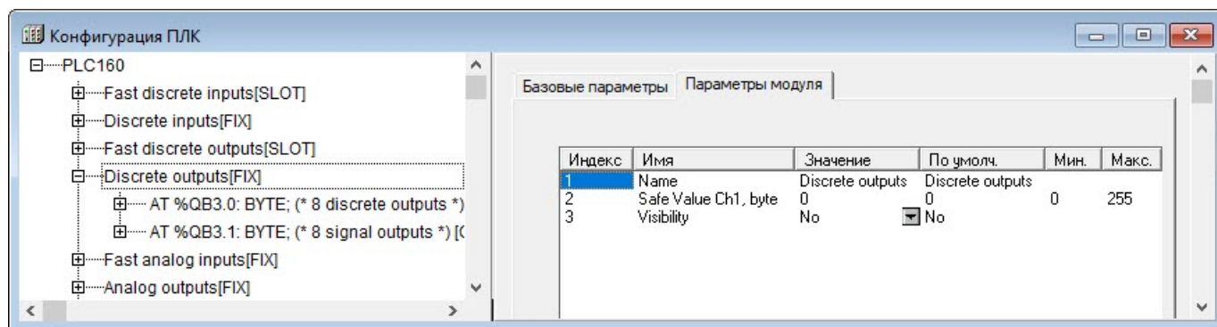
Рисунок 10.20 – Параметры модуля Дискретные выходы (Discrete outputs)
