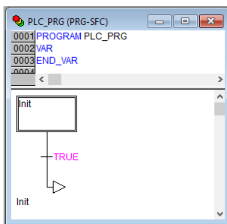
Рисунок 6.13 – Пример программы на языке SFC
