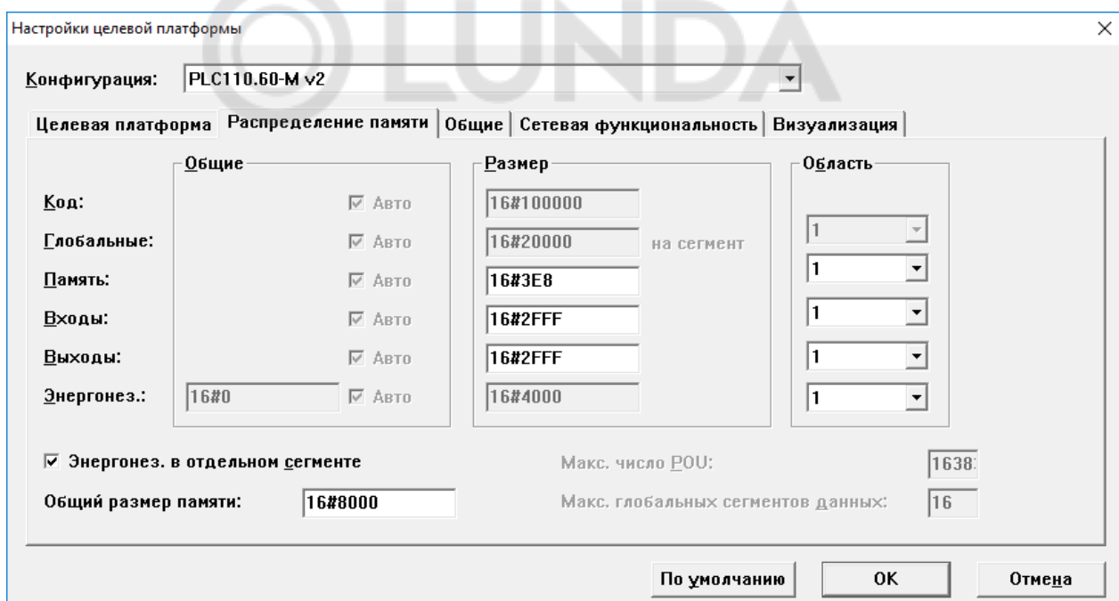
Рисунок 6.4 – Увеличение размера памяти входов-выходов на вкладке «Распределение памяти» (Memory Layout)
