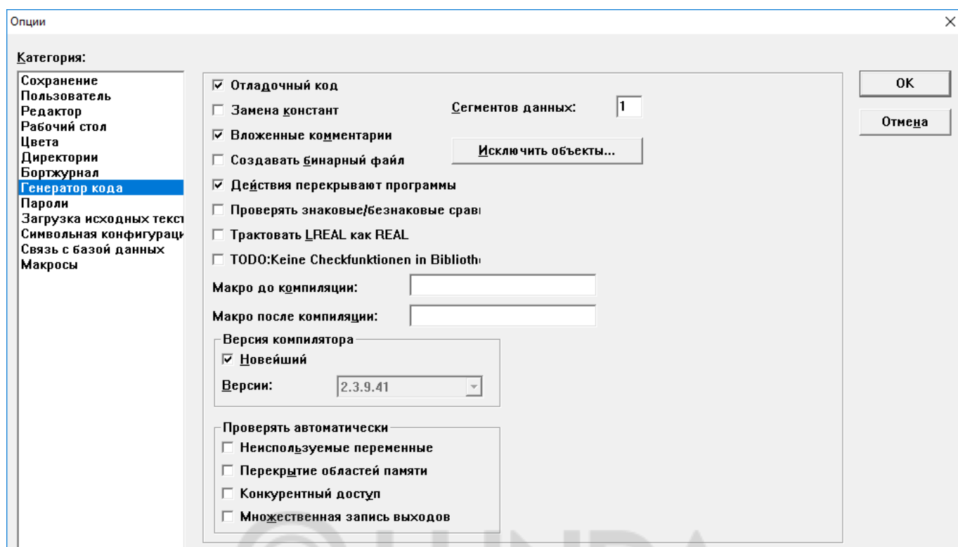
Рисунок 7.27 – Окно «Опции...», вкладка «Генератор кода»
