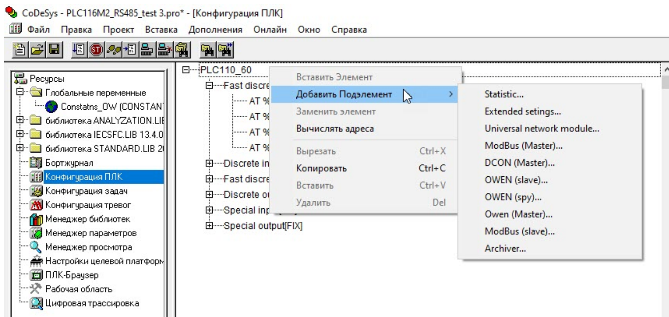
Рисунок 10.5 – Добавление подмодуля в контекстном меню
