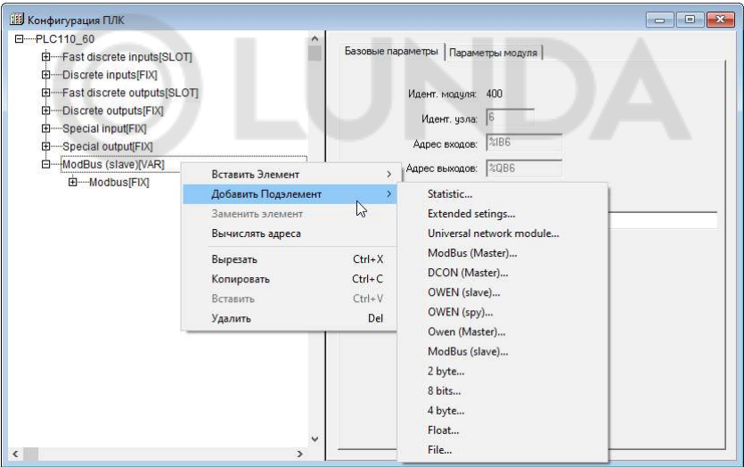
Рисунок 10.31 – Добавление переменных в модуль «ModBus (Slave)»
