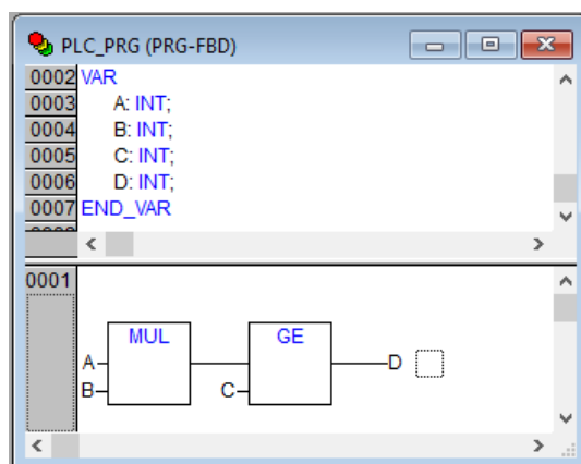
Рисунок 6.11 – Пример программы на языке FBD
