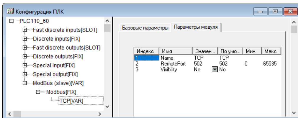
Рисунок 10.58 – Параметры порта TCP
