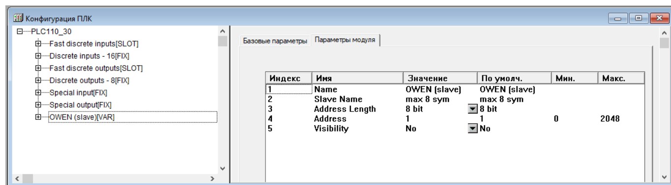
Рисунок 10.39 – Параметры модуля «Owen (Slave)»
