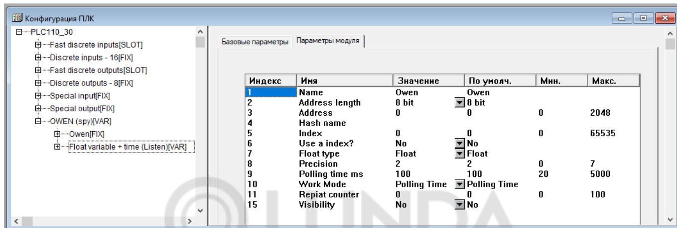
Рисунок 10.47 – Параметры переменных протокола ОВЕН
