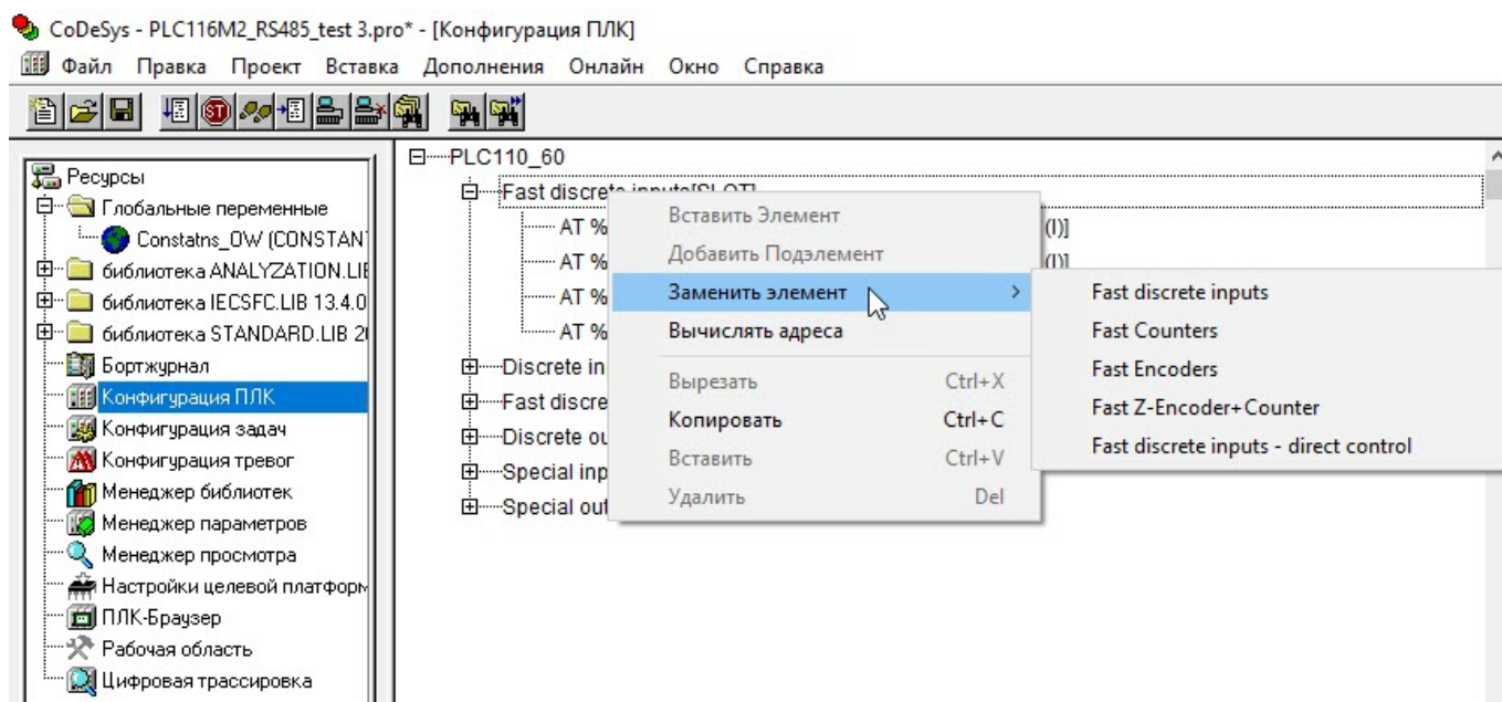
Рисунок 10.6 – Замена элемента в контекстном меню
