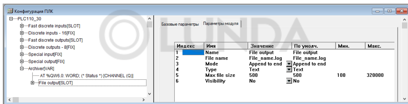
Рисунок 10.54 – Параметры подмодуля «File output»
