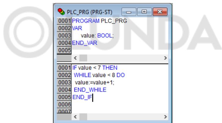
Рисунок 6.10 – Пример программы на языке ST
