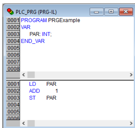
Рисунок 7.1 – Пример записи программы на языке IL
