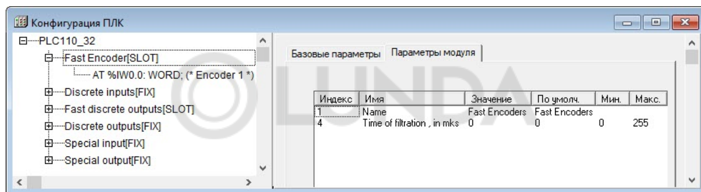
Рисунок 10.13 – Параметры модуля Высокочастотный энкодер (FastEncoder) для ПЛК110-32
