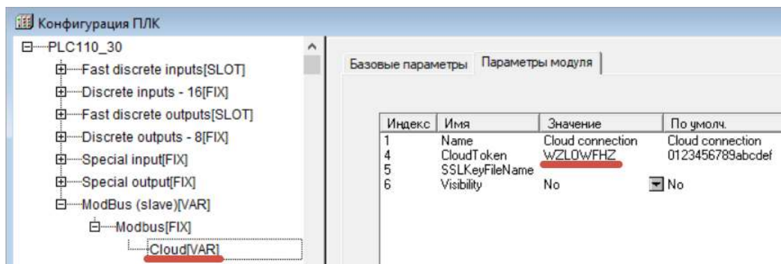
Рисунок 13.9 – Ввод токена OwenCloud в конфигурацию ПЛК
