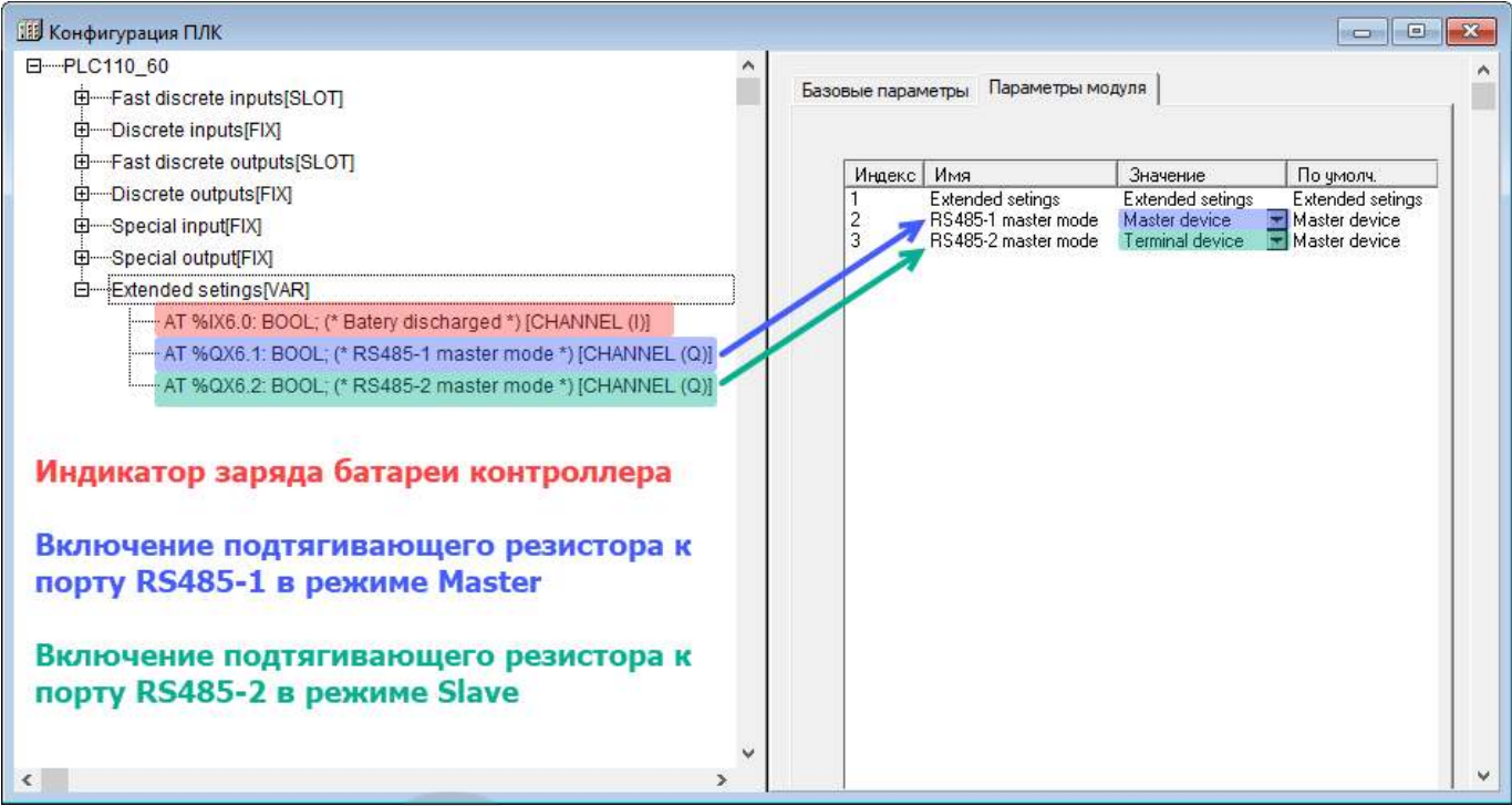
Рисунок 10.55 – Параметры модуля «Extended settings»
