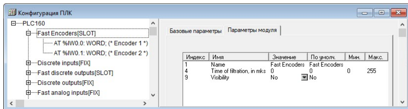
Рисунок 10.14 – Параметры модуля Высокочастотный энкодер (FastEncoder) для ПЛК160
