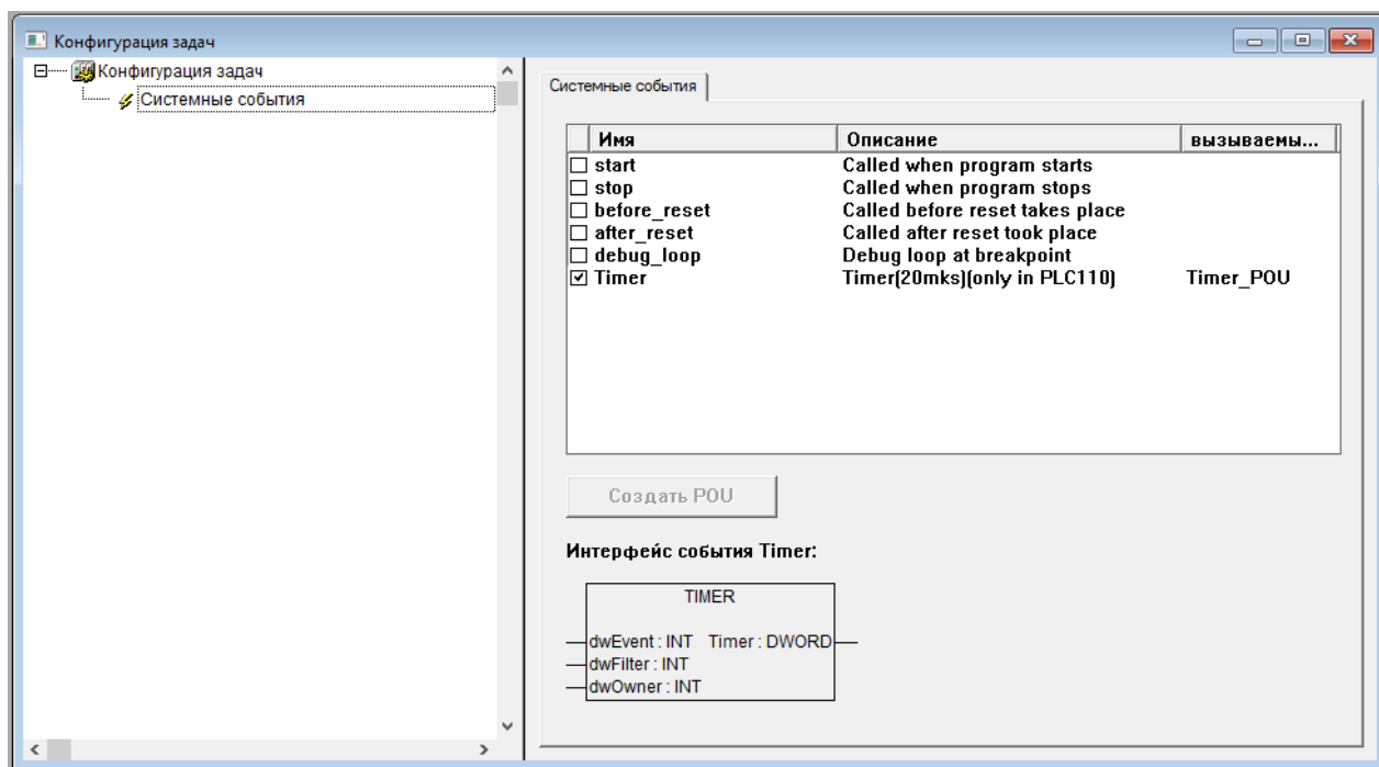
Рисунок 14.2 – Окно режима «Конфигурация задач» (Task Configuration)
