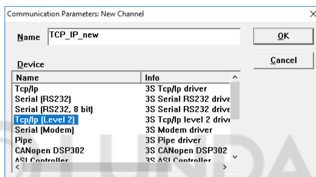
Рисунок 6.18 – Создание нового TCP/IP соединения
