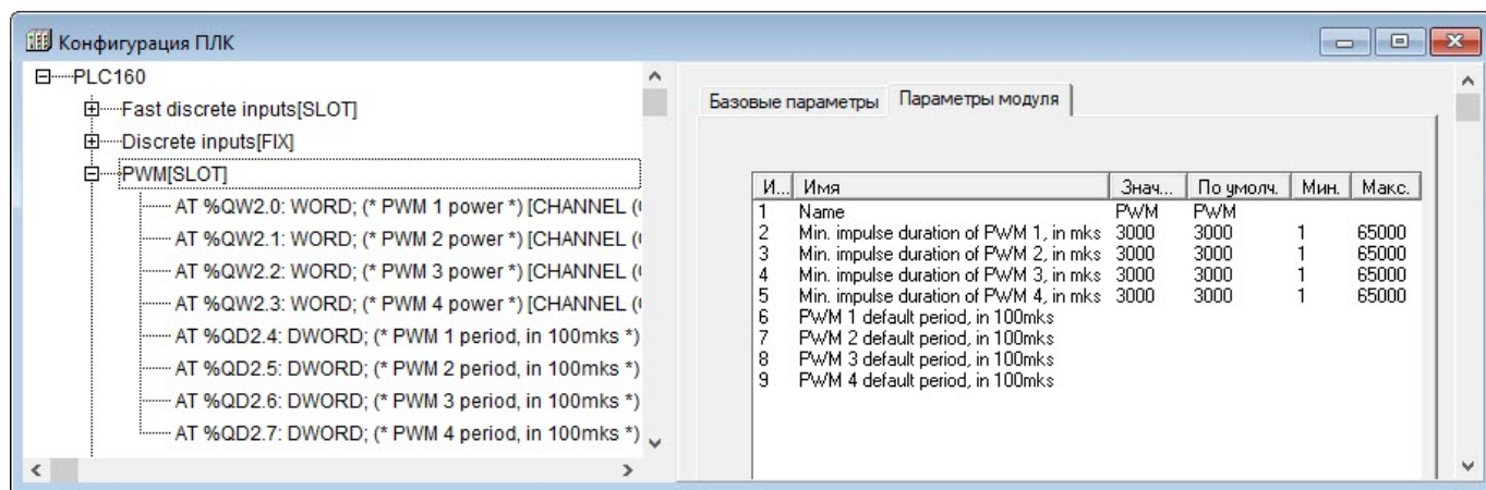
Рисунок 10.19 – Параметры модуля ШИМ (PWM – Pulse-wide modulator)
