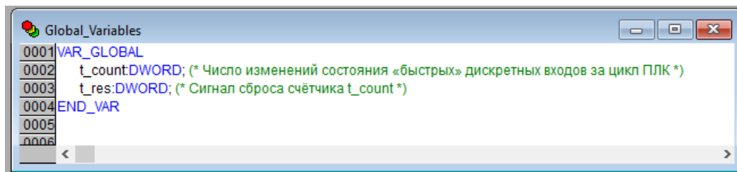
Рисунок 14.6 – Глобальные переменные, используемые программой обработки высокочастотного таймера («Timer_POU»)
