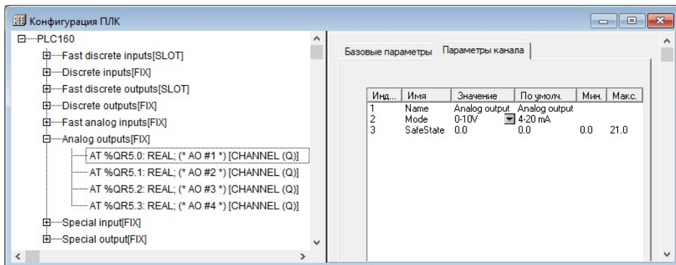
Рисунок 10.22 – Параметры модуля аналогового выхода
