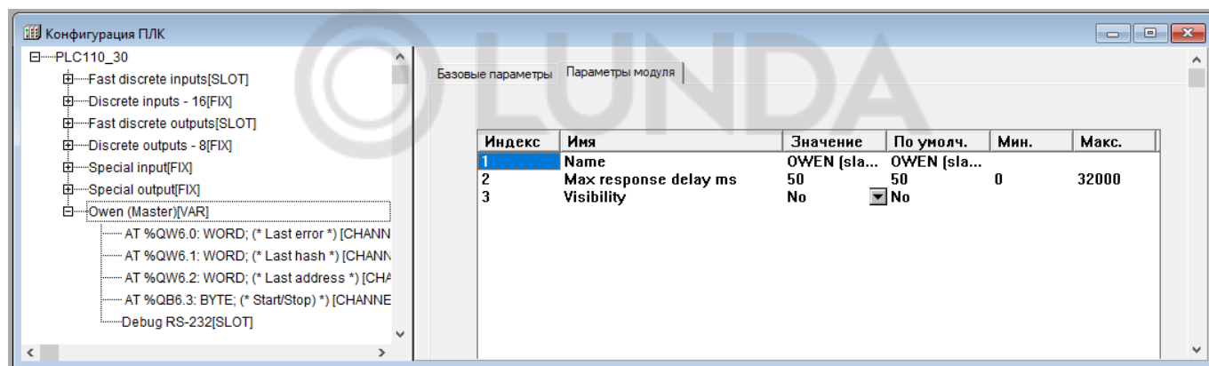
Рисунок 10.35 – Каналы и параметры модуля «Owen (Master)»
