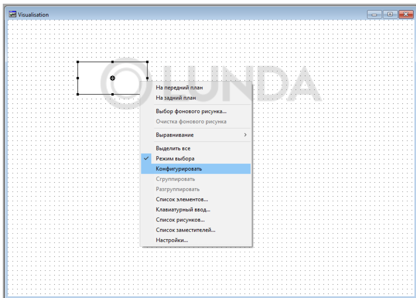
Рисунок 9.1 – Контекстное меню элемента визуализации
