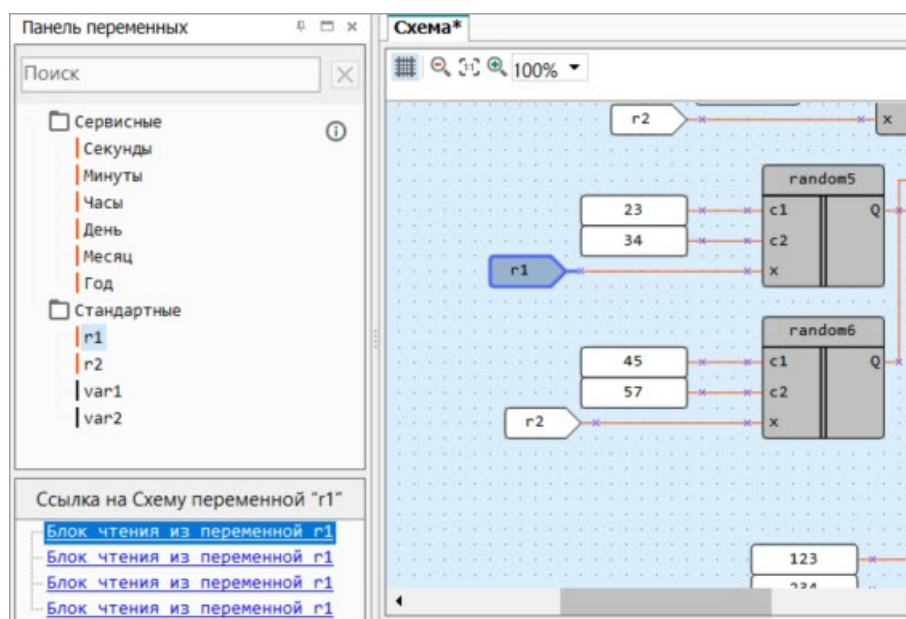
Рисунок 3.8 – Ссылка на переменную
