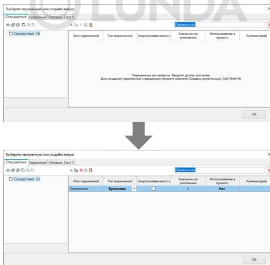
Рисунок 6.4 – Создание переменной с заданным именем
