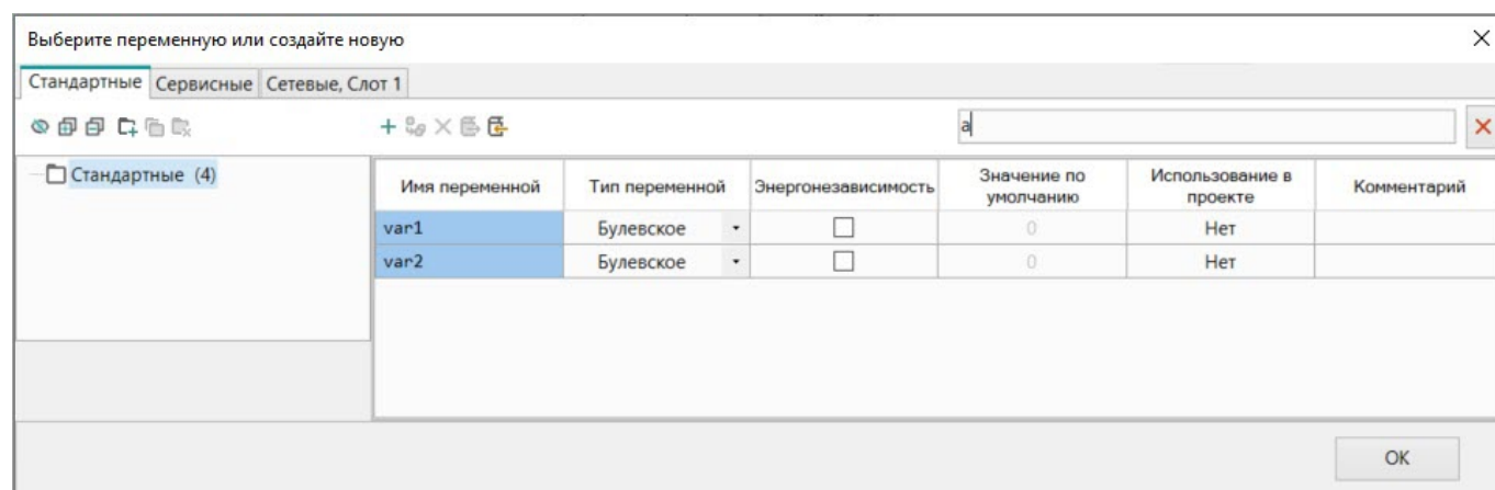
Рисунок 6.3 – Поиск переменных
