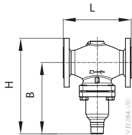
VFG-2R DN15-125
