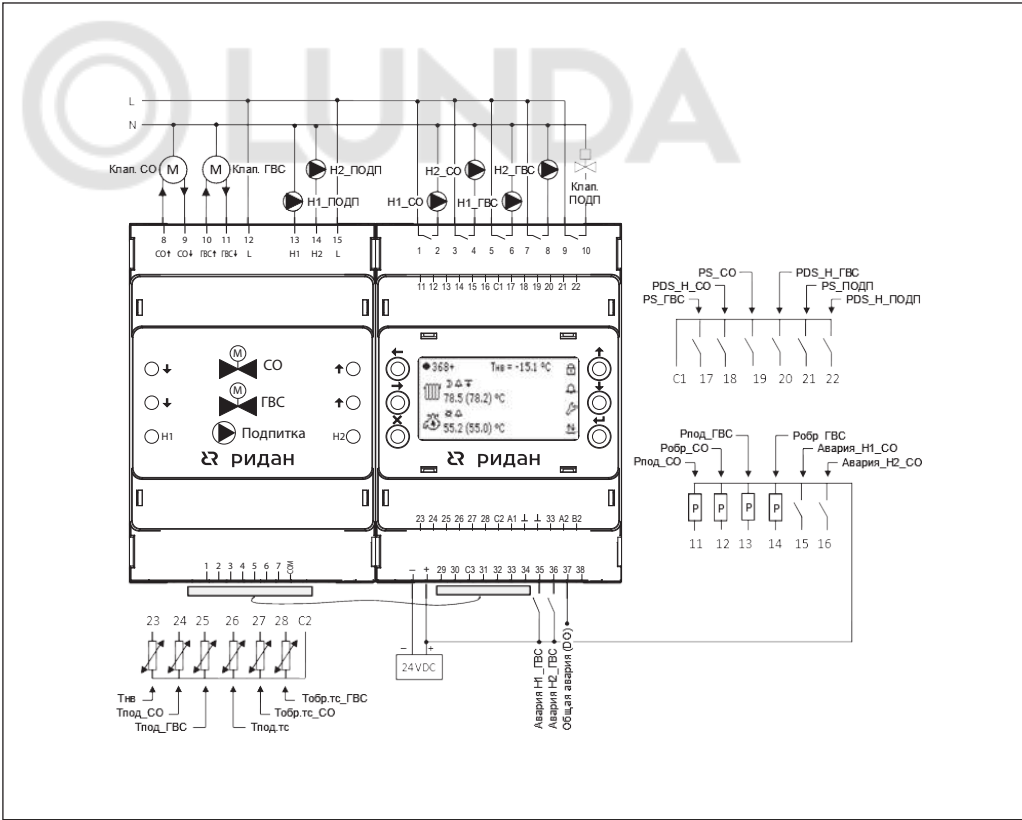
Схема электрических подключений ECL-3R 368
