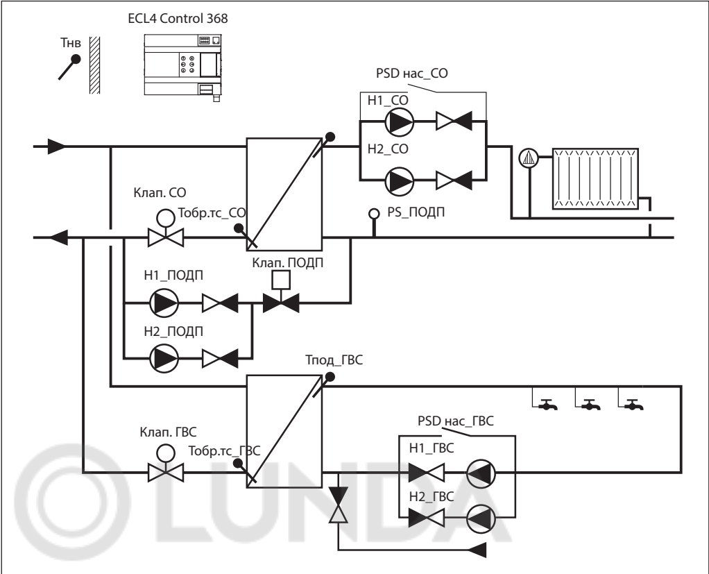
Схема приложения для ECL4 Control 368R и ECL4 Control 368R Ethernet
