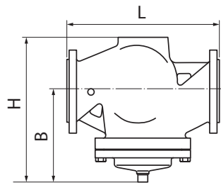
VFG-2R DN150-250
