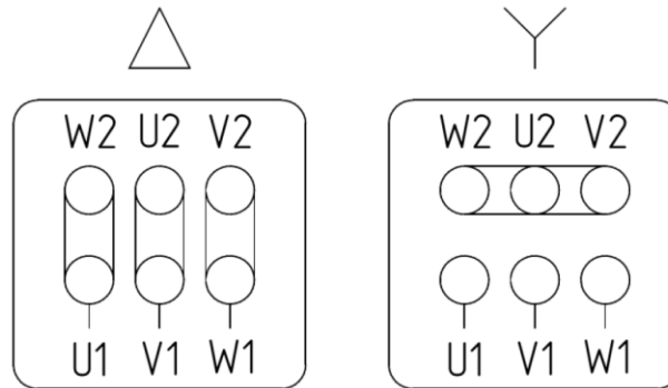
Рис. 9 Схема клеммных соединений
