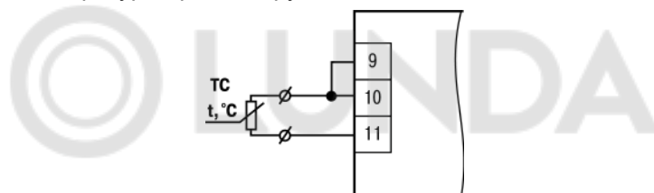
Рисунок 5.5 – Подключение ТС по двухпроводной схеме
