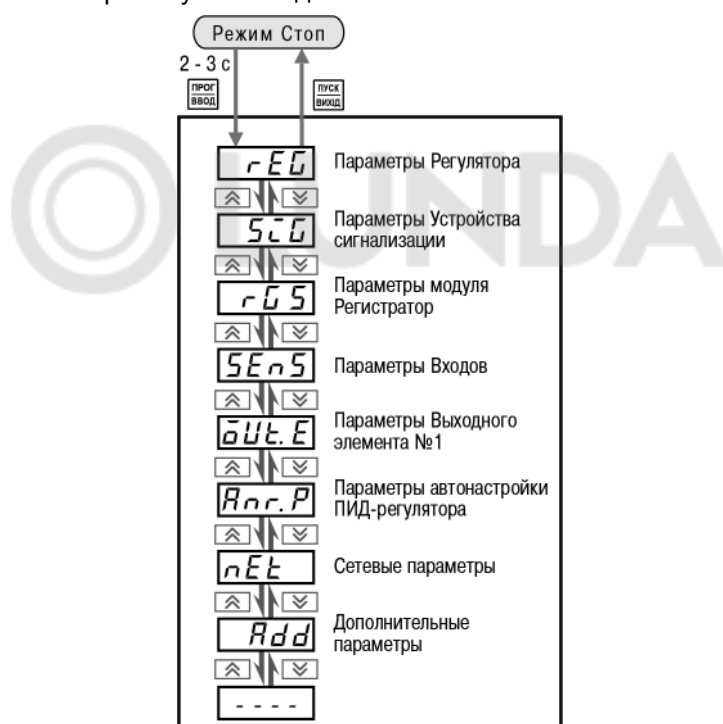
Рисунок 8.2 – Главное меню прибора
