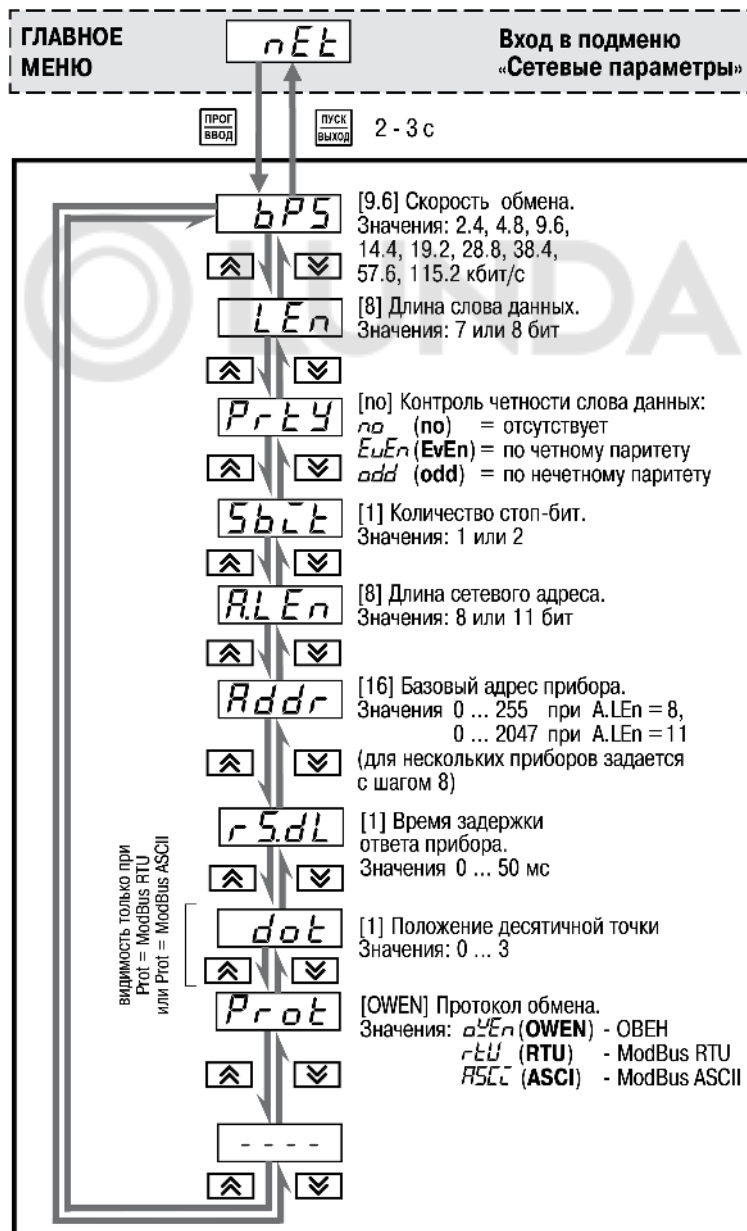
Рисунок 8.9 – Сетевых параметров
