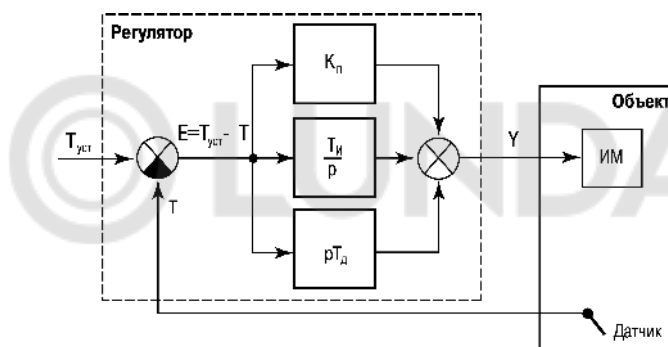
Рисунок 7.7 – Структурная схема ПИД-регулятора
