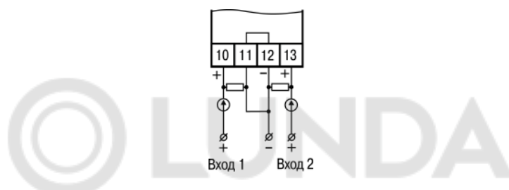
Рисунок 5.6 – Подключение активных датчиков
