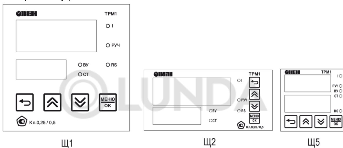
Рисунок 6.2 – Лицевая панель
