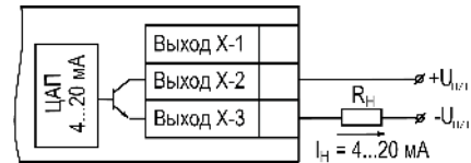
Рисунок 5.22 – Подключение к ВУ типа «И»
