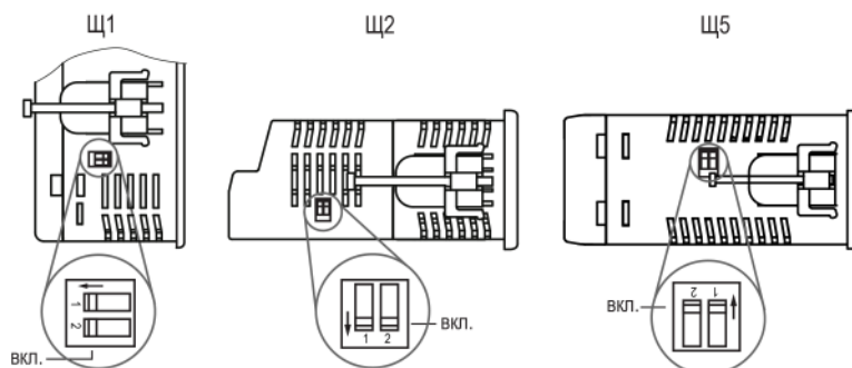
Рисунок 5.15 – Расположение DIP-переключателей
