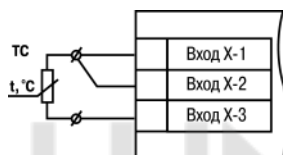
Рисунок 5.10 – Трехпроводная схема подключения ТС
