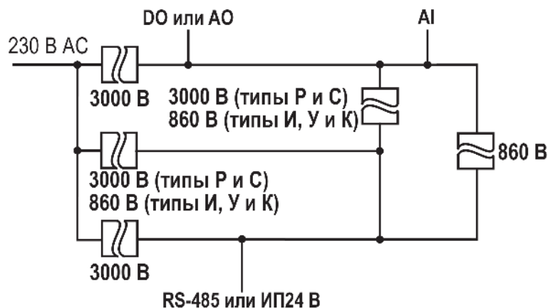
Рисунок 5.3 – Схема гальванической развязки (выходы кроме типа «Т»)
