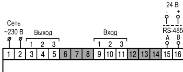
Рисунок 5.7 – Общая схема подключения ТРМ1–Н
