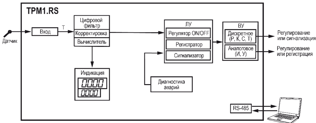
Рисунок 6.1 – Функциональная схема
