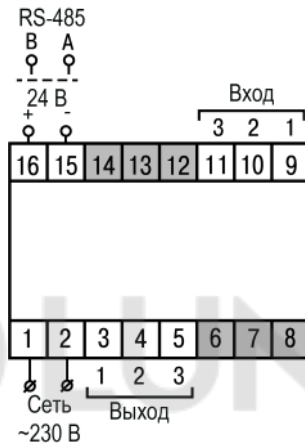
Рисунок 5.6 – Общая схема подключения ТРМ1–Д
