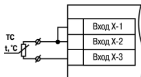
Рисунок 5.11 – Двухпроводная схема подключения ТС
