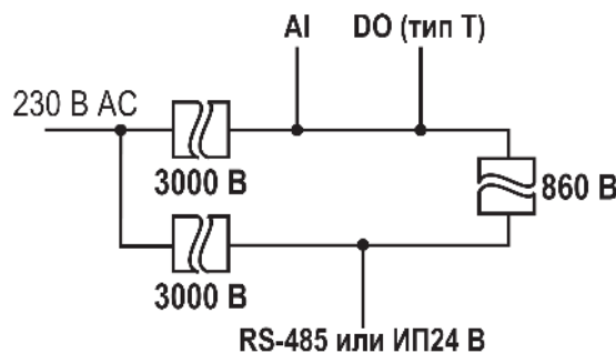
Рисунок 5.2 – Схема гальванической развязки (выход типа «Т»)
