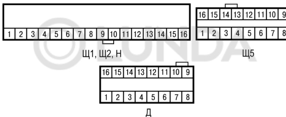
Рисунок 7.9 – Установка переключки
