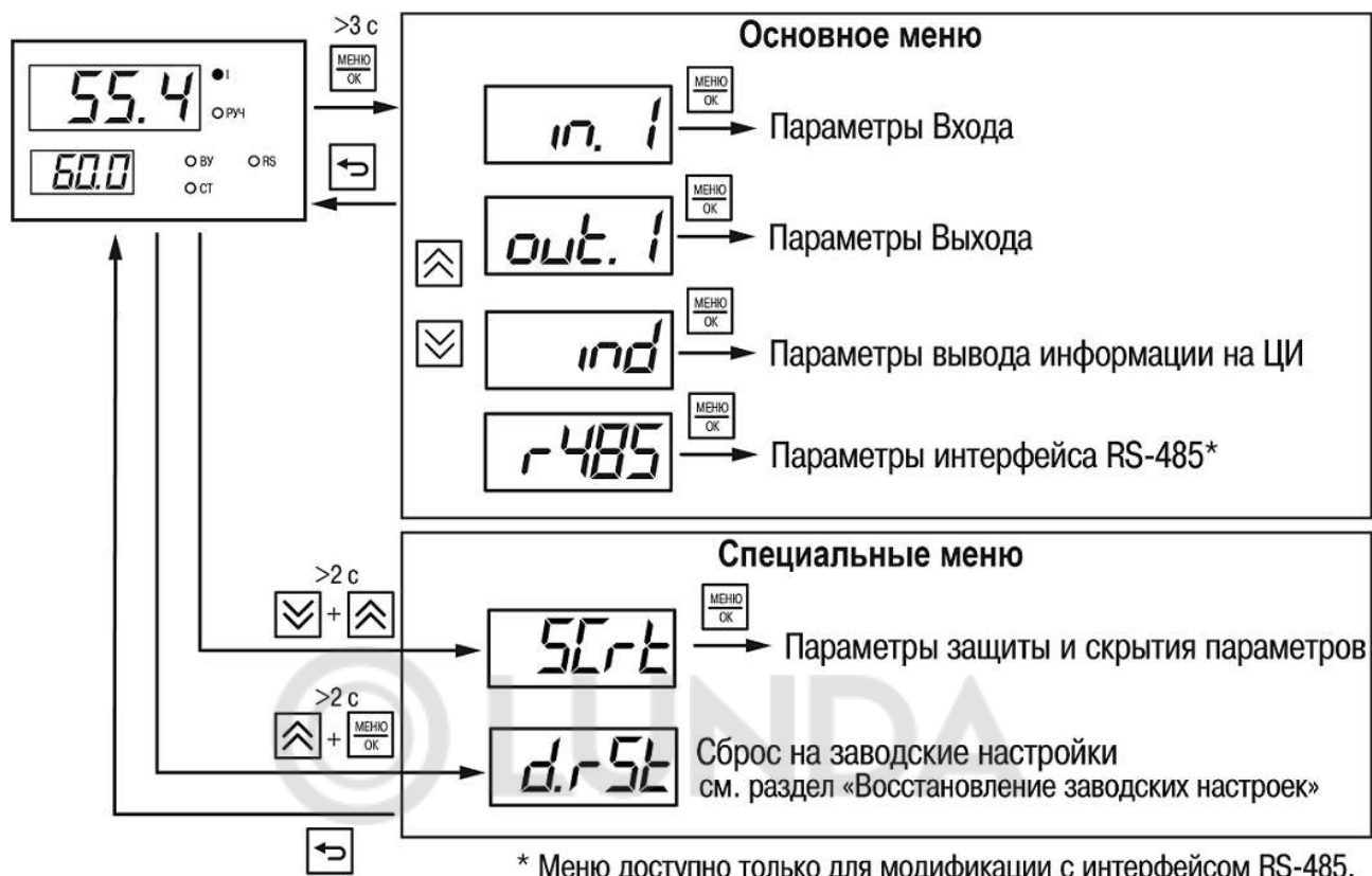
Рисунок 7.1 – Структура меню
