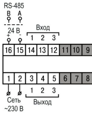
Рисунок 5.5 – Общая схема подключения ТРМ1–Ц5
