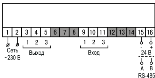
Рисунок 5.4 – Общая схема подключения ТРМ1–Щ1/Щ2
