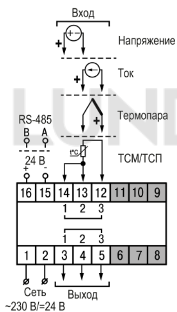
Рисунок 5.5 – Общая схема подключения ТРМ1–Ц5
