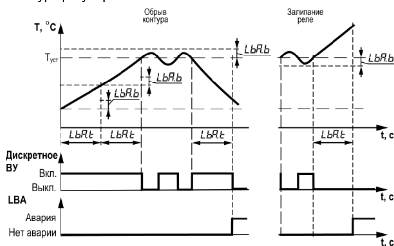
Рисунок 7.5 – Принцип работы диагностики обрыва в контуре регулирования
