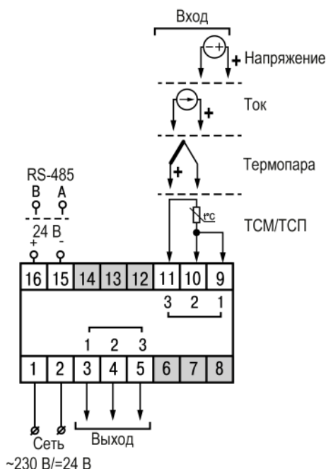
Рисунок 5.6 – Общая схема подключения ТРМ1-Д
