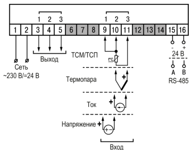
Рисунок 5.4 – Общая схема подключения ТРМ1–Ц1/Ц2
