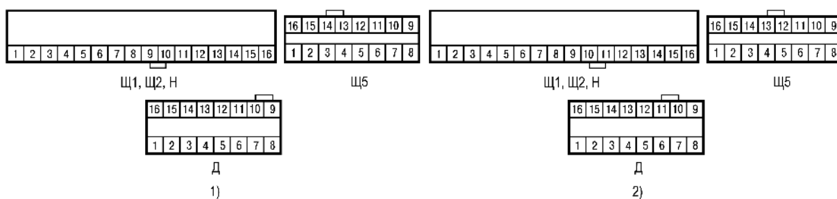
Рисунок 7.9 – Установка перемычки
