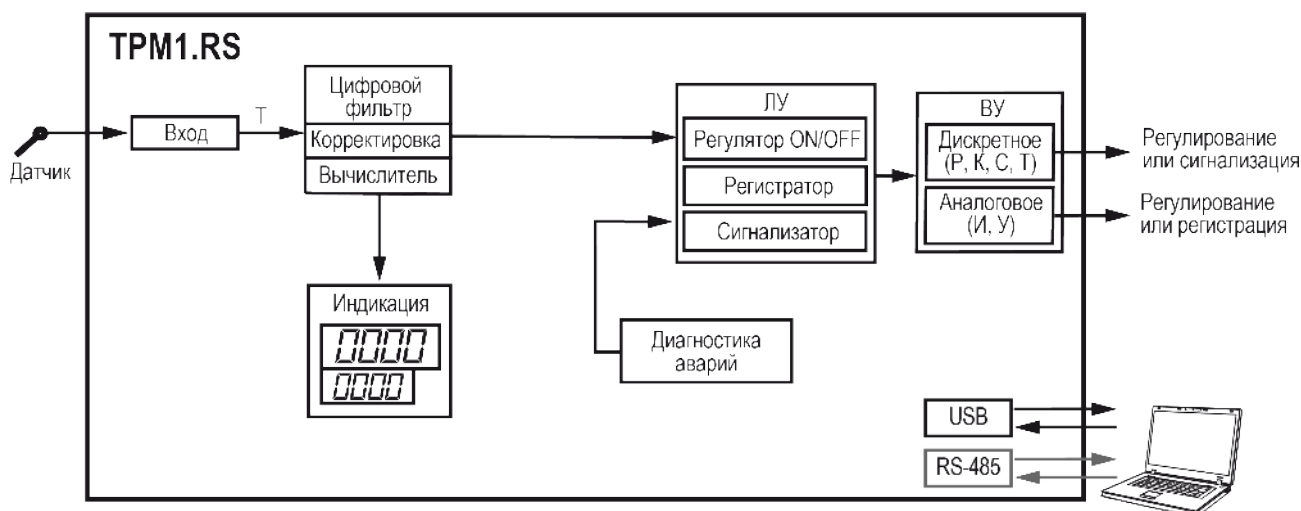
Рисунок 6.1 – Функциональная схема
