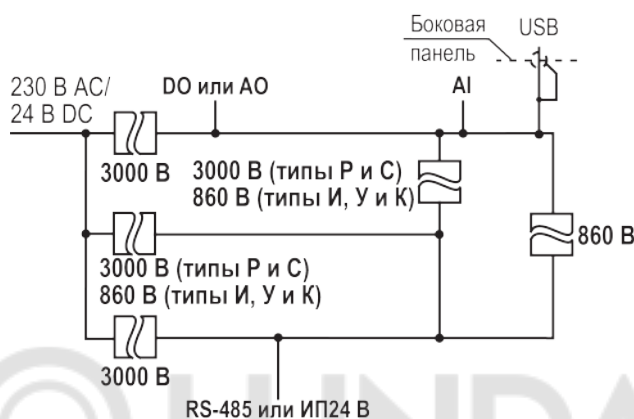
Рисунок 5.3 – Схема гальванической развязки (выходы кроме типа «Т»)
