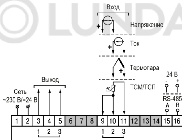
Рисунок 5.7 – Общая схема подключения ТРМ1-Н
