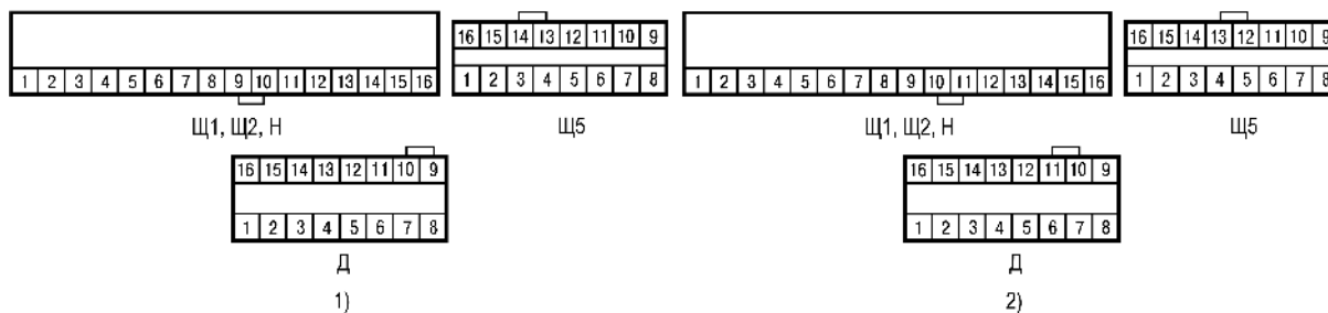
Рисунок 7.8 – Установка переключки
