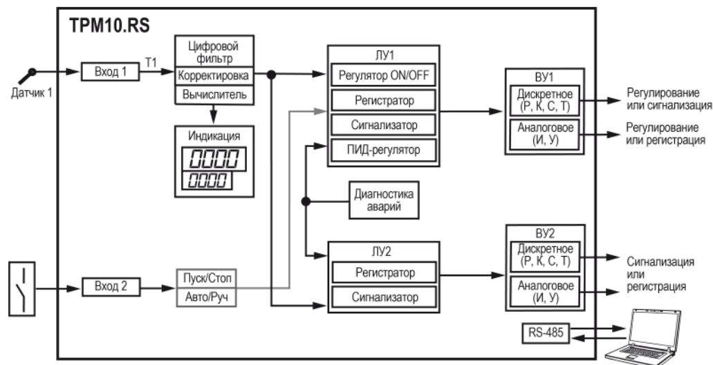
Рисунок 6.1 – Функциональная схема
