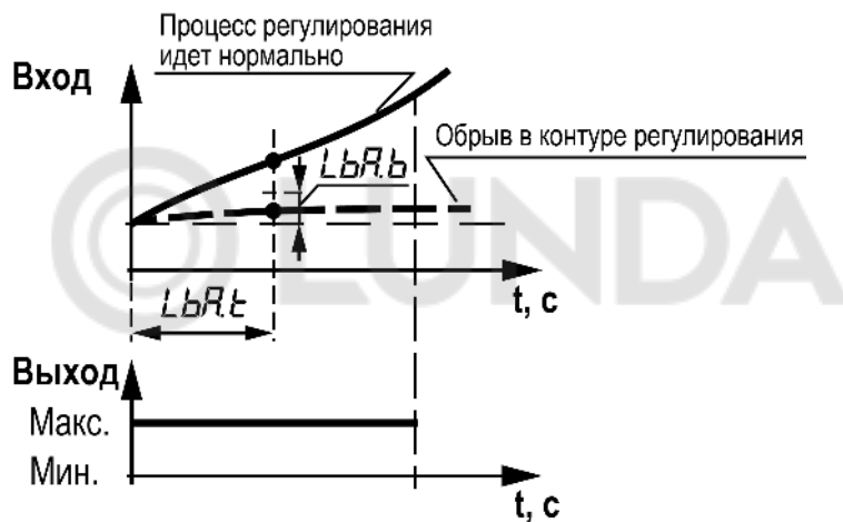
Рисунок 7.4 – Диагностика неисправности контура регулирования
