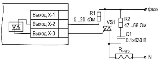
Рисунок 5.21 – Схема подключения силового симистора к ВУ типа «С»
