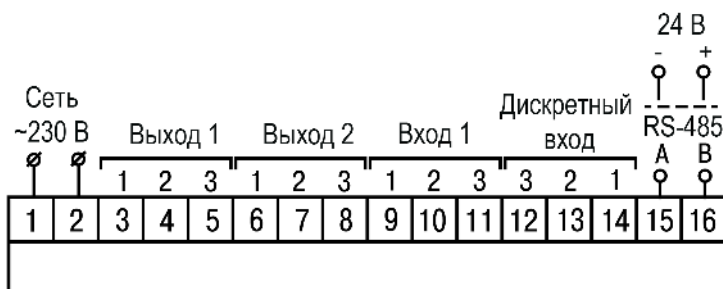
Рисунок 5.7 – Общая схема подключения TRM10–Н
