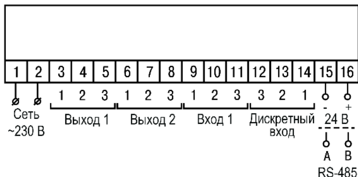
Рисунок 5.4 – Общая схема подключения ТРМ10–Щ1/Щ2
