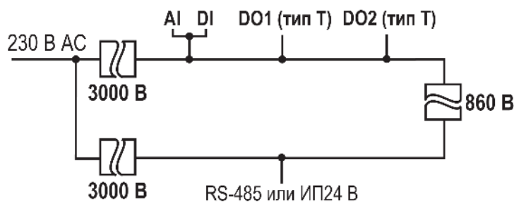
Рисунок 5.2 – Схема гальванической развязки (выход типа «Т»)
