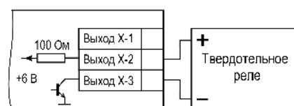
Рисунок 5.20 – Схема подключения нагрузки к ВУ типа «Т»
