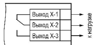
Рисунок 5.18 – Схема подключения нагрузки к ВУ типа «Р»
