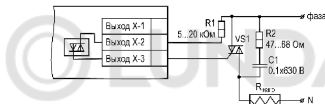
Рисунок 5.25 – Схема подключения силового симистора к ВУ типа «С»
