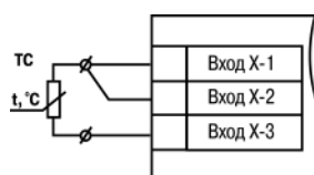
Рисунок 5.16 – Трехпроводная схема подключения ТС
