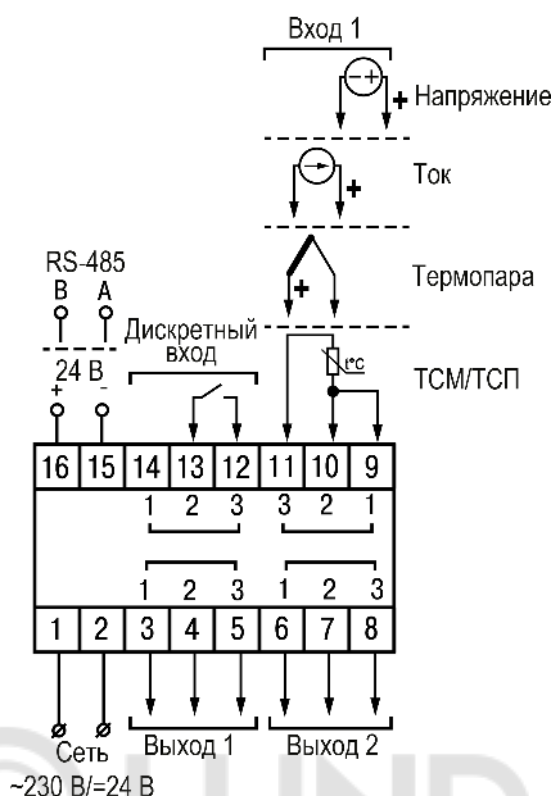
Рисунок 5.6 – Общая схема подключения ТРМ10–Д
