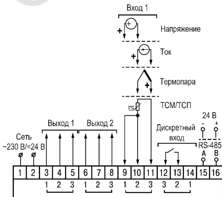
Рисунок 5.7 – Общая схема подключения ТРМ10–Н
