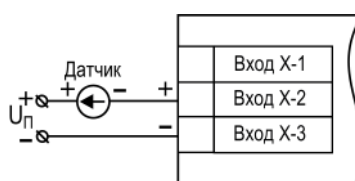
Рисунок 5.21 – Схема подключения пассивного датчика с выходным сигналом силы постоянного тока от 0 до 5 мА или от 0(4) до 0 мА
