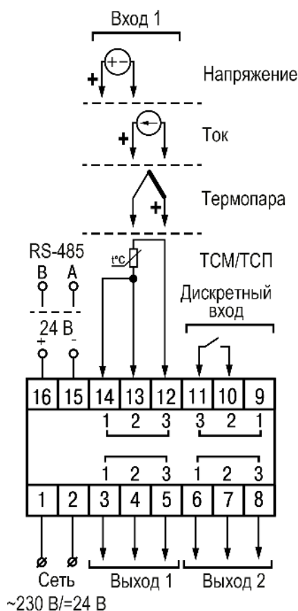
Рисунок 5.5 – Общая схема подключения TRM10–Щ5
