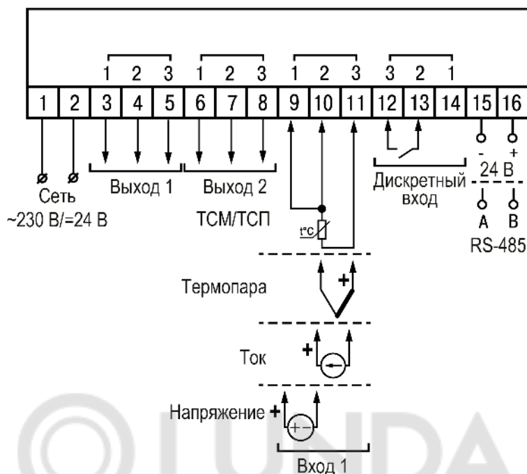
Рисунок 5.4 – Общая схема подключения TRM10–Щ1/Щ2
