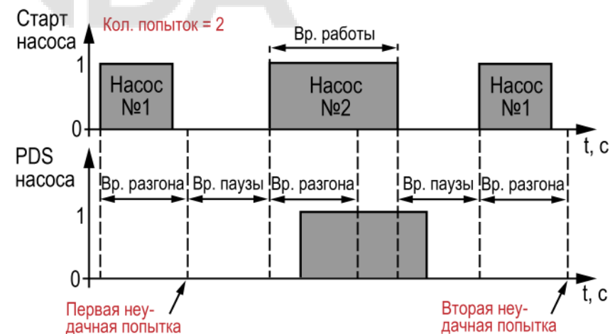
Рисунок 14.8 – Перезапуск насоса
