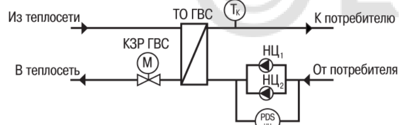
Рисунок 3.2 – Схема контура «ГВС»
