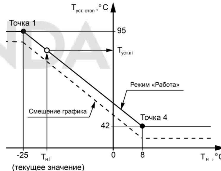
Рисунок 13.3 – Отопительный график
