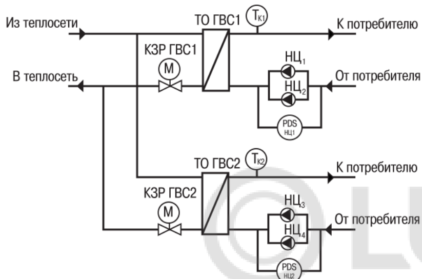
Рисунок 3.5 – Схема контура «ГВС + ГВС»
