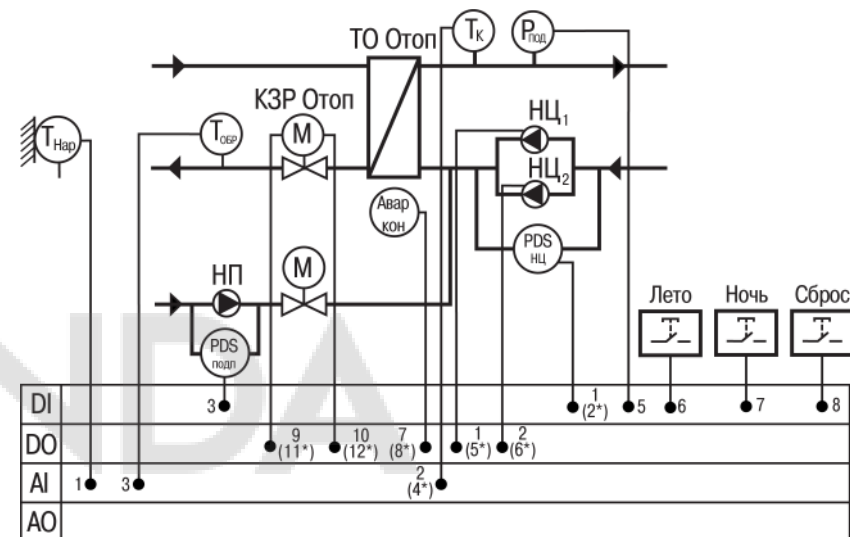
Рисунок 4.1 – Функциональная схема контура «Отопление»
