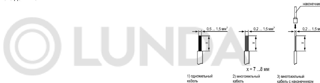
Рисунок 9.1 – Требования к сечениям жил кабелей
