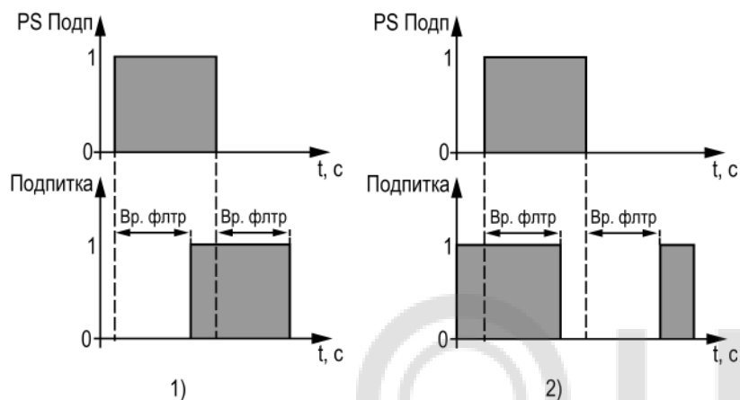
Рисунок 11.6 – Логика работы реле давления: 1) НО, 2) НЗ
