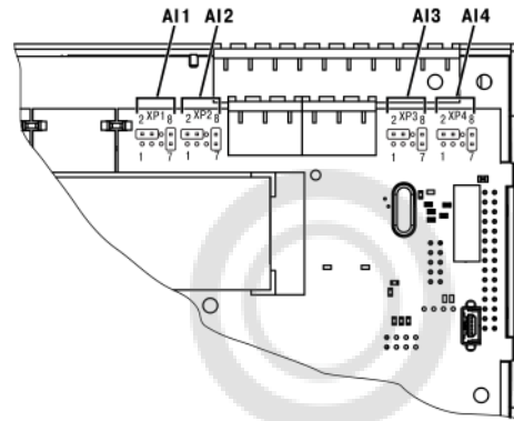
Рисунок 8.3 – Расположение входов
