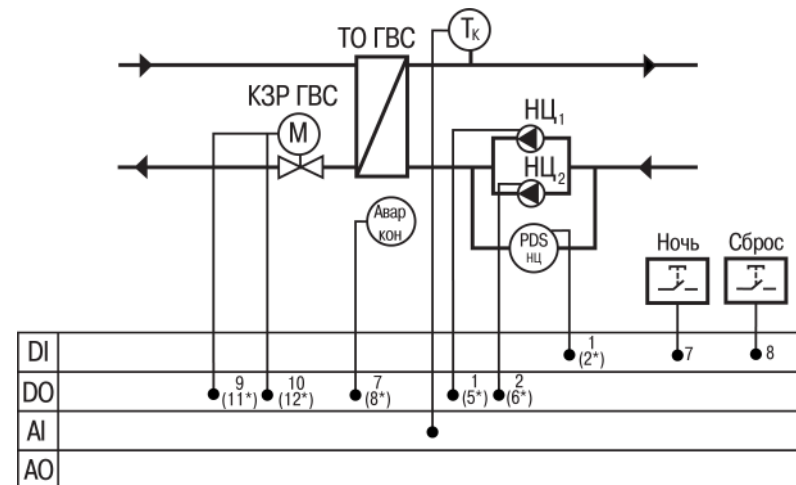
Рисунок 4.2 – Функциональная схема контура «ГВС»
