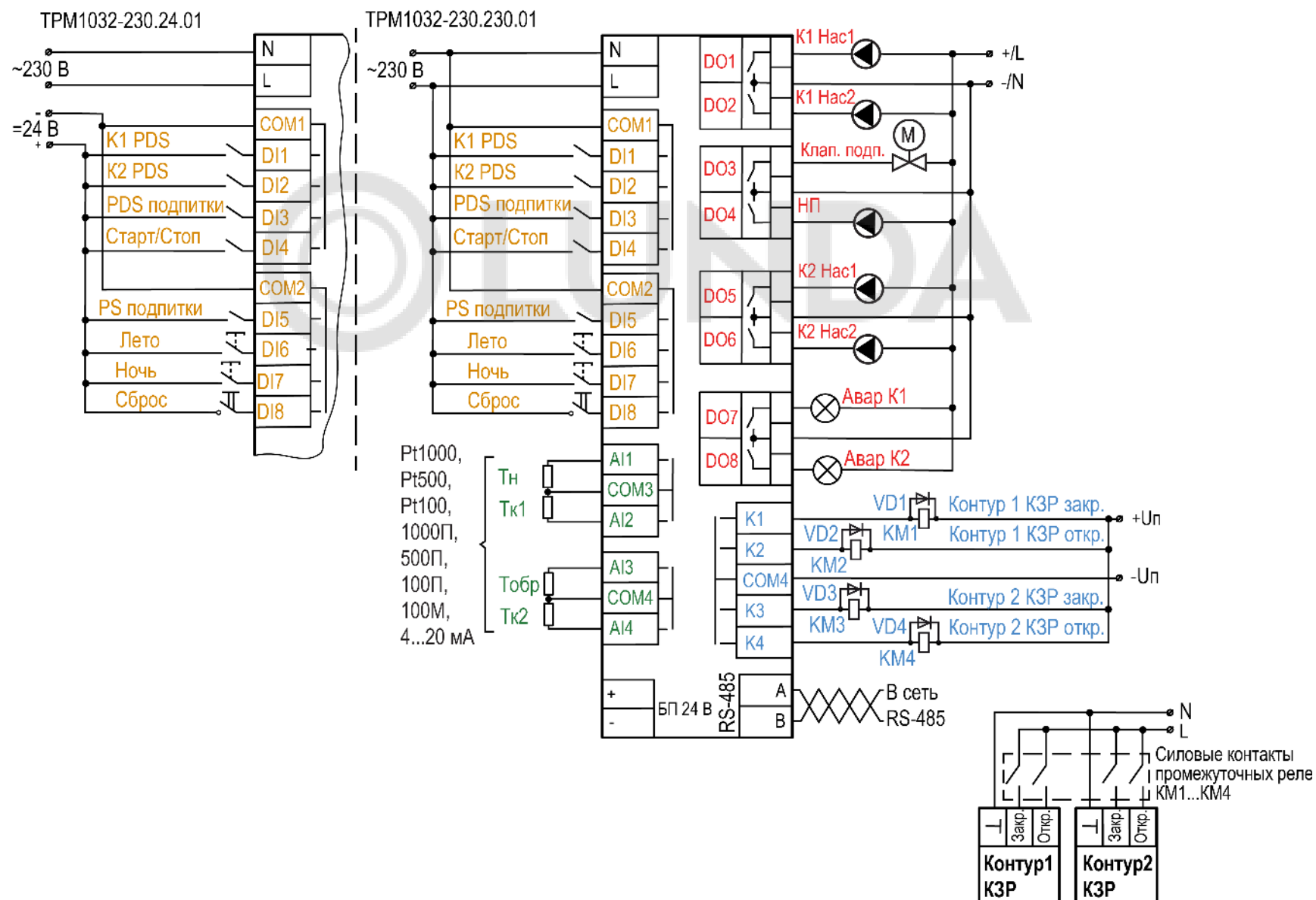
Рисунок 9.3 – Схема подключения
