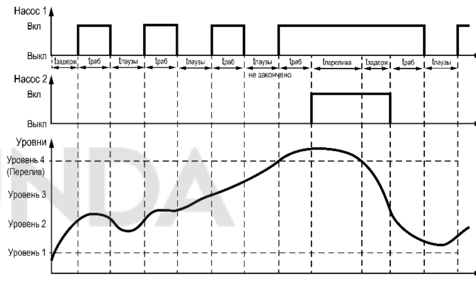
Рисунок 8.6 – Авария аналогового датчика уровня
