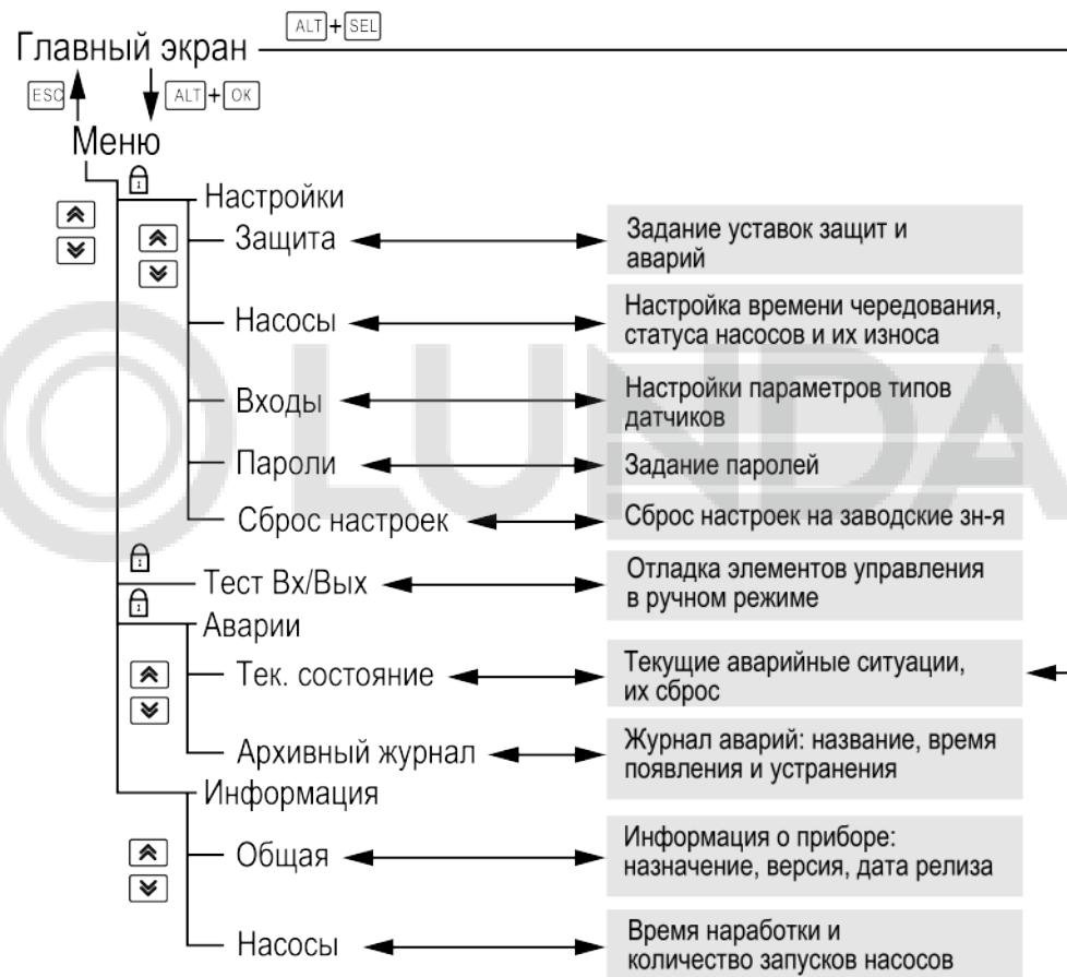
Рисунок 6.2 – Схема переходов по меню
