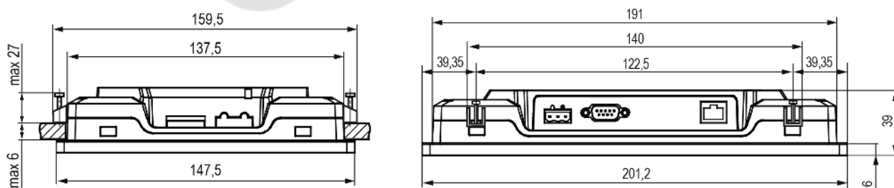
Рисунок 4.3 – Дополнительные установочные размеры СПК210-07
