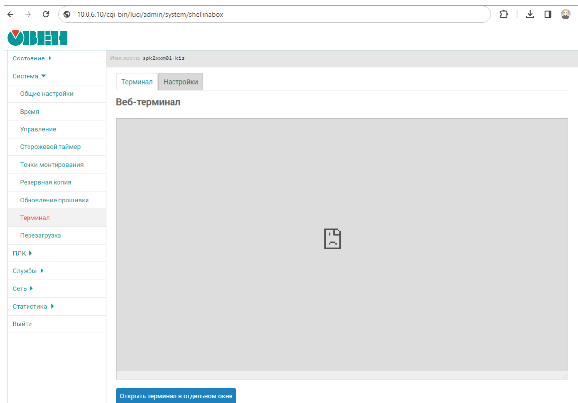
Рисунок 6.4 – Страница «Терминал»
