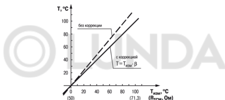
Рисунок 7.7 – Коррекция «наклон характеристики»
