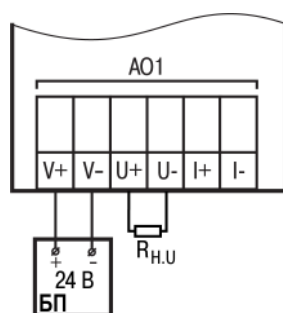
Рисунок 5.12 – Схема подключения нагрузки типа У
