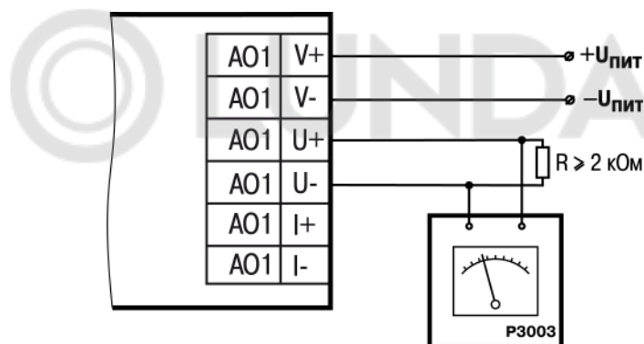
Рисунок А.9 – Схема подключения нагрузки к ВЭ типа У
