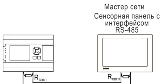
Рисунок 6.17 – Типовая схема подключения в режиме Slave
