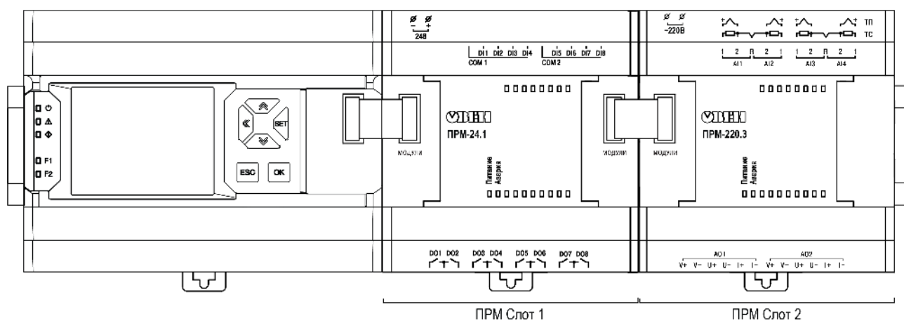
Рисунок 6.16 – Расположение модулей расширения на шине
