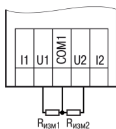
Рисунок 6.10 – Подключение резистивных датчиков
