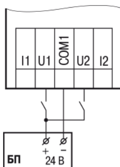
Рисунок 6.5 – Схема подключения к универсальным входам, работающим в дискретном режиме датчиков типа «сухой» контакт
