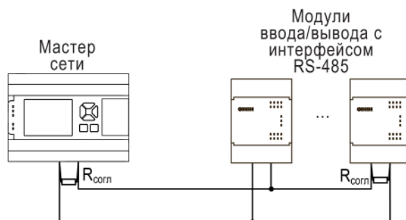
Рисунок 6.18 – Типовая схема подключения в режиме Master
