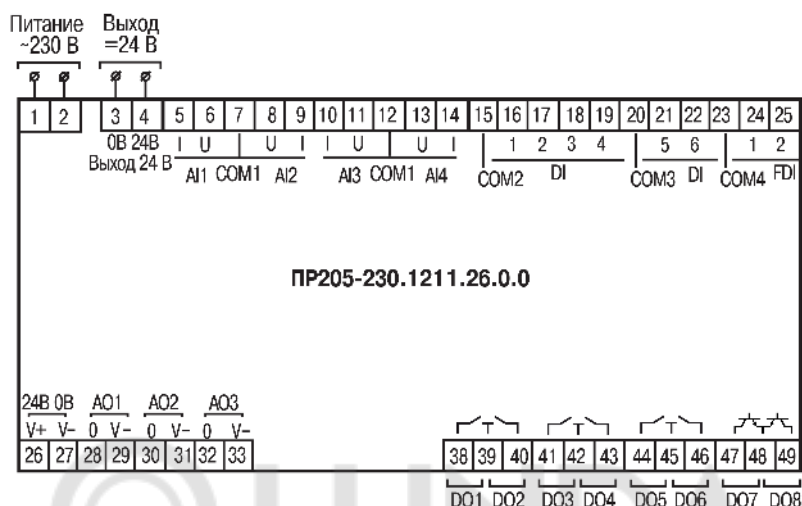
Рисунок А.3 – Расположение контактов для ПР205-230.1211.26.0.0
