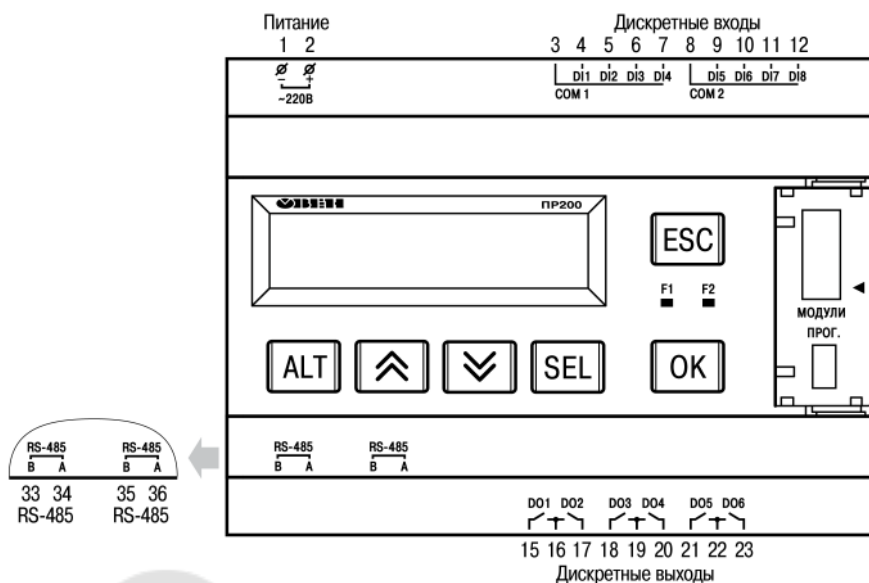
Рисунок А.1 – Расположение контактов ПР200-220.1.2.Х
