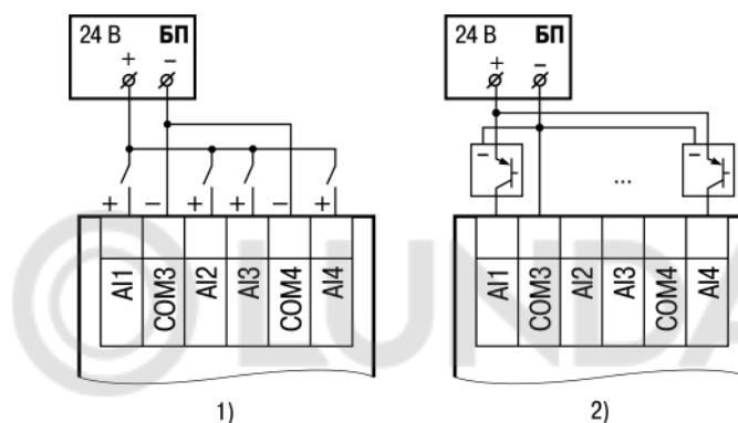
Рисунок 6.8 – Схема подключения к аналоговым входам, работающим в дискретном режиме: 1) датчиков типа «сухой» контакт, 2) трехпроводных дискретных датчиков, имеющих выходной транзистор р-п-р-типа с открытым коллектором
