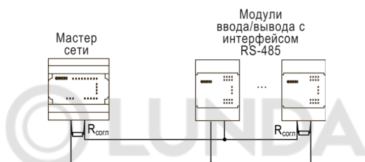
Рисунок 6.10 – Типовая схема подключения для ПР100 в режиме Master
