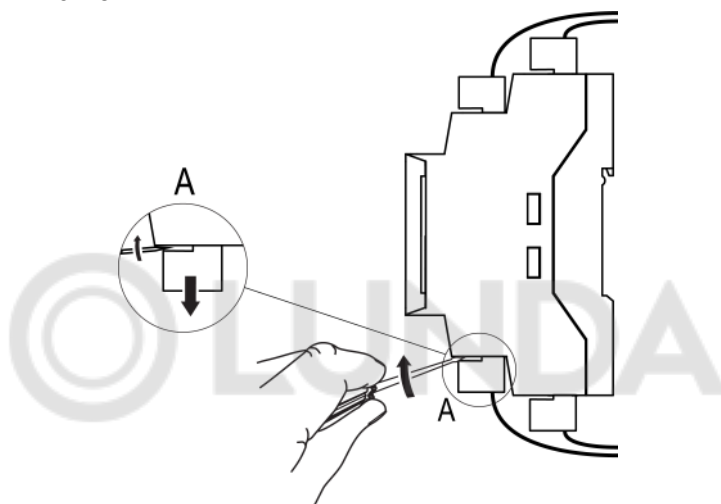
Рисунок 5.3 – «Быстрая» замена прибора
