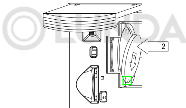
Рисунок 3.7 – Установка новой батареи
