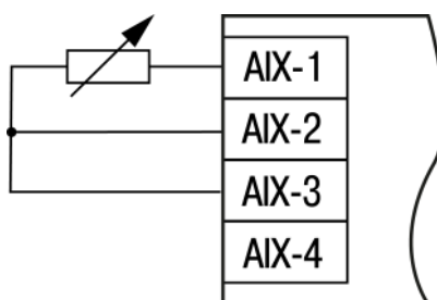
Рисунок 5.20 – Схема подключения датчиков типа 0\dots 2 кОм и 0\dots 5 кОм
