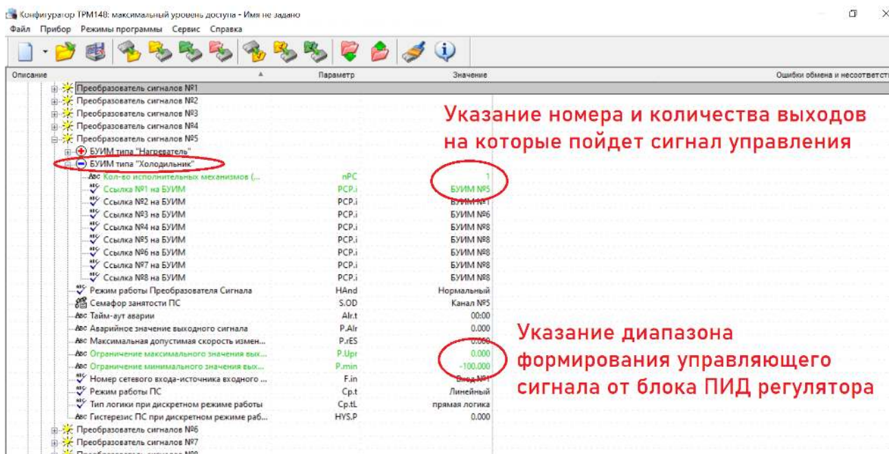
Рисунок 2.11 – Настройка логики Холодильник. В папке БУИМ типа Нагреватель параметр nPC должен быть равен нулю
