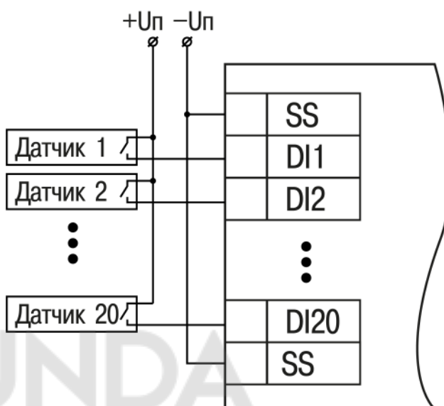
Рисунок 5.5 – Схема подключения к входам DI1–DI20 – вариант 2 (MB210-202)
