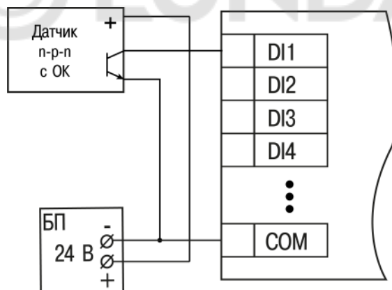
Рисунок 5.9 – Подключение транзисторов п-р-п (MB210-204)
