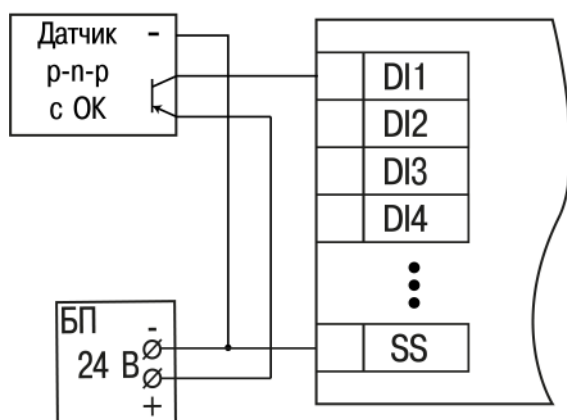
Рисунок 5.7 – Подключение транзисторов р-п-р (MB210-202)
