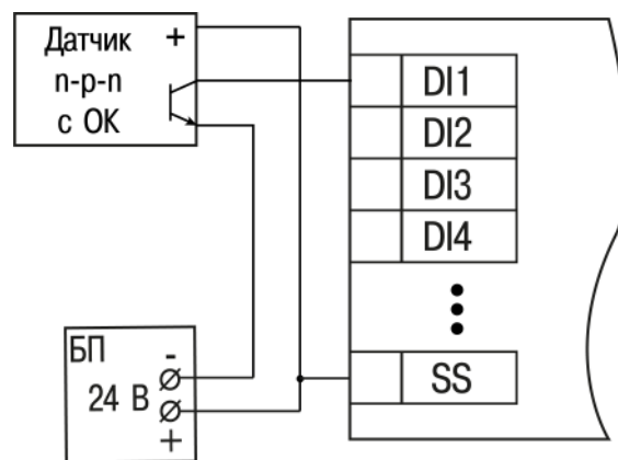
Рисунок 5.8 – Подключение транзисторов п-р-п (MB210-202)
