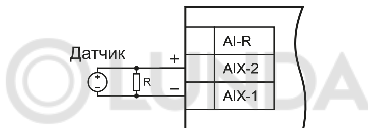
Рисунок 8.1 – Подключение резистора (R = 10 кОм)
