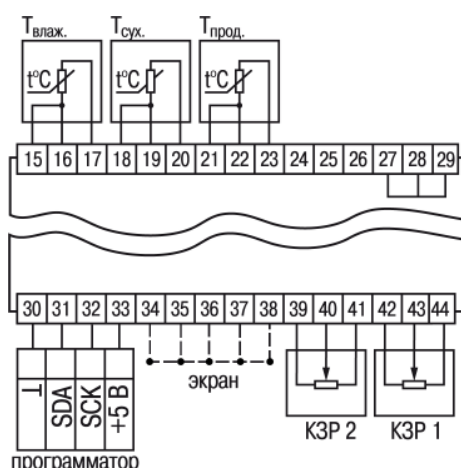
Рисунок 5.3 – Подключение измерительных датчиков и датчиков положения задвижек
