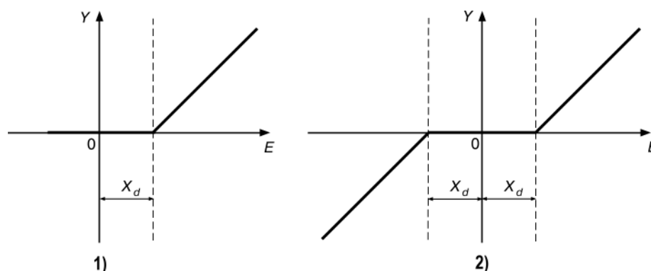
Рисунок 7.17 – 1) Зона нечувствительности для исполнительного устройства типа «нагреватель» 2) Зона нечувствительности для исполнительного устройства типа «нагреватель – холодильник» или «здвижка»
