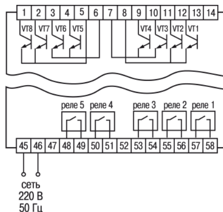
Рисунок 5.4 – Схема подключения транзисторных ключей и выходных устройств
