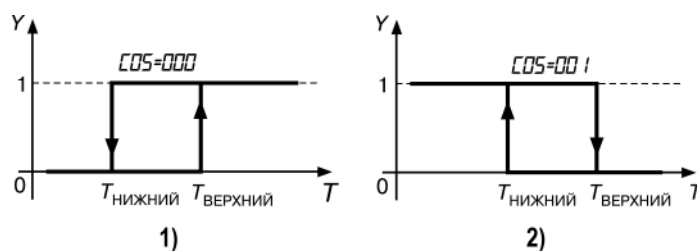
Рисунок 7.18 – 1) Компаратор срабатывает по верхней уставке: Y = 1 — выходное реле замкнуто, Y = 0 — выходное реле разомкнуто 2) Компаратор срабатывает по нижней уставке: Y = 1 — выходное реле замкнуто, Y = 0 — выходное реле разомкнуто
