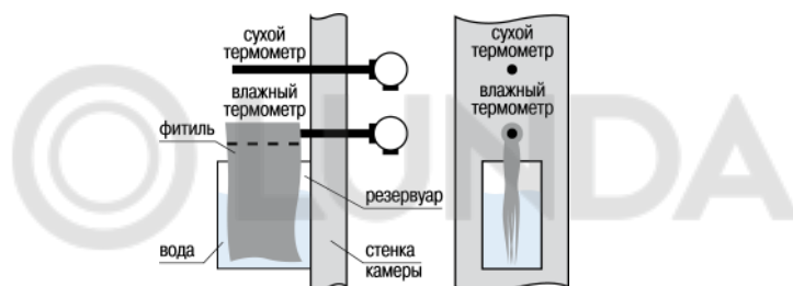
Рисунок Б.1 – Крепление датчиков температуры перпендикулярно стенке камеры
