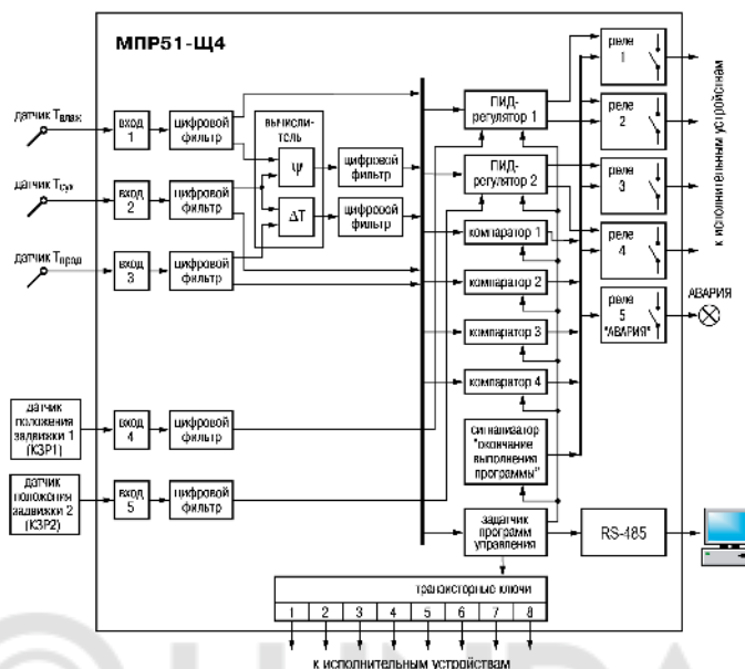
Рисунок 6.1 – Функциональная схема прибора
