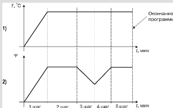
Рисунок 7.10 – Определение общего числа шагов : 1) программа первого регулятора 2) программа второго регулятора
