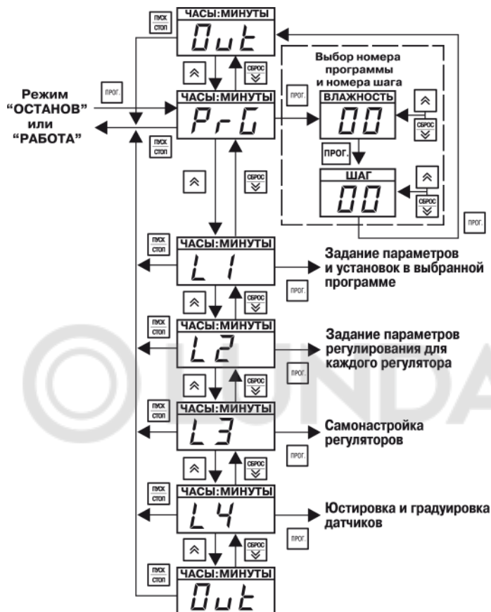
Рисунок 7.2 – Основное меню
