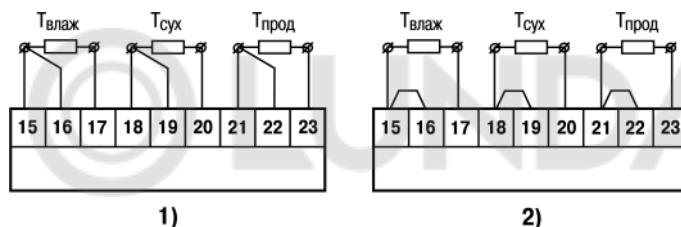
Рисунок 5.5 – Соединение датчиков по: 1) трехпроводной схеме, 2) двухпроводной схеме
