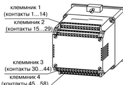
Рисунок 5.2 – Назначение контактов клеммника
