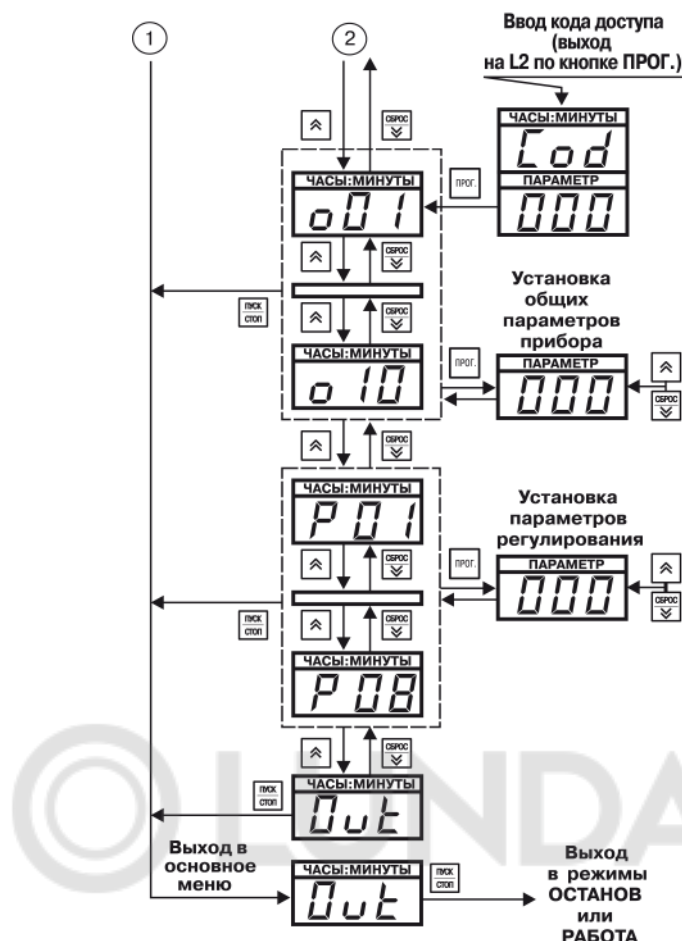
Рисунок 7.6 – Схема настройки на уровне L2 (конец)
