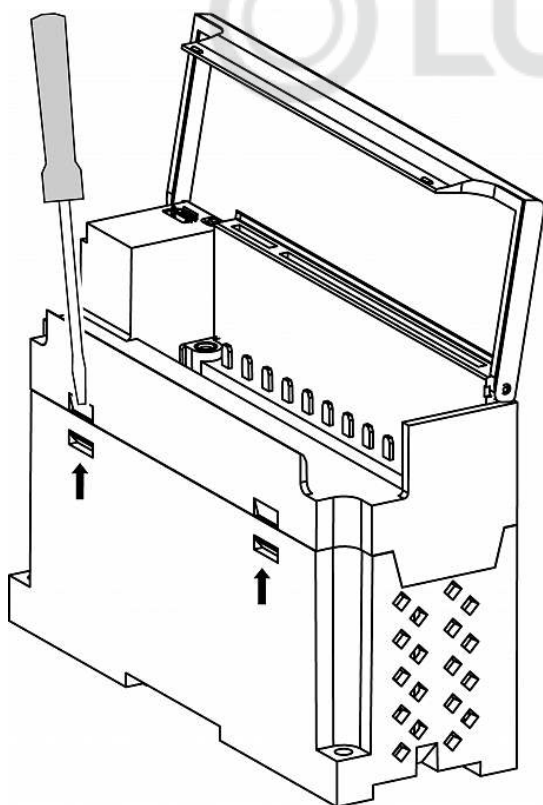
Рисунок 8.2 – Замена батареи
