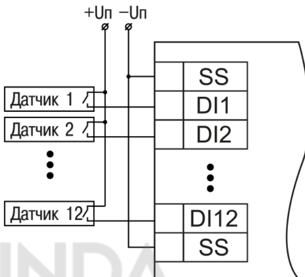
Рисунок 5.5 – Схема подключения к входам DI1-DI12 – вариант 2
