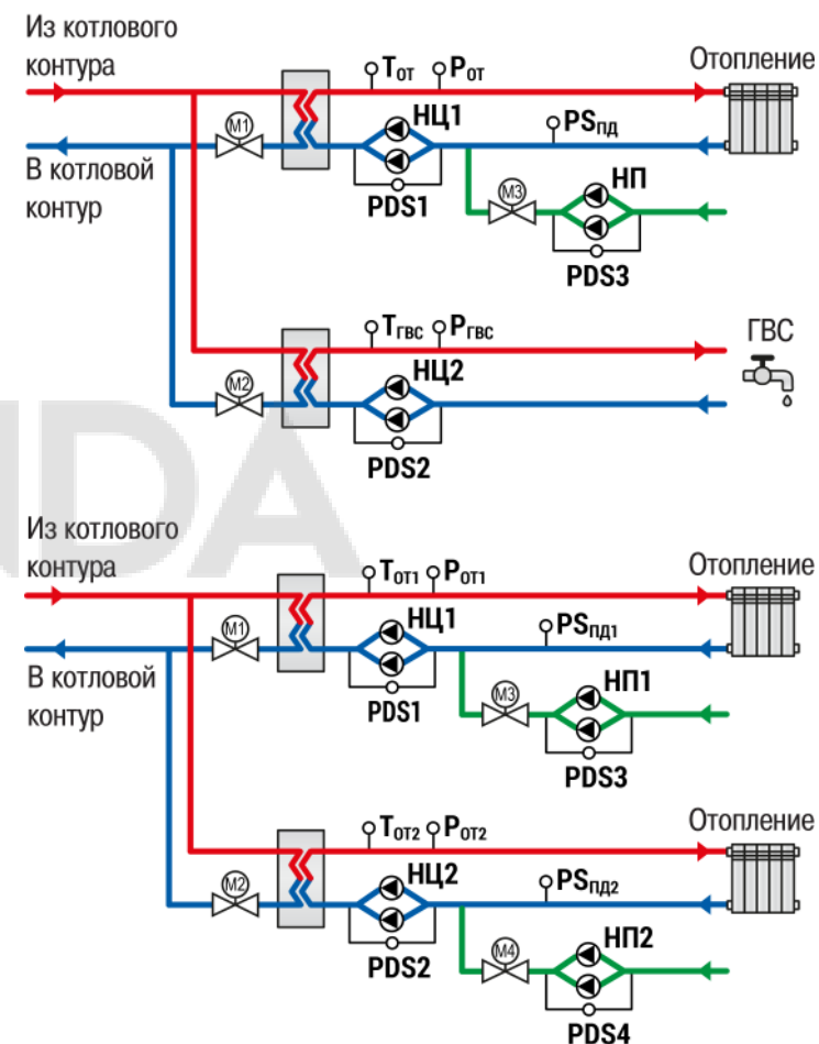
Рисунок 1.2 – Схемы управления контурами ГВС и отопления с подпиткой при использовании КТР-121.03.20 и ПРМ-1
