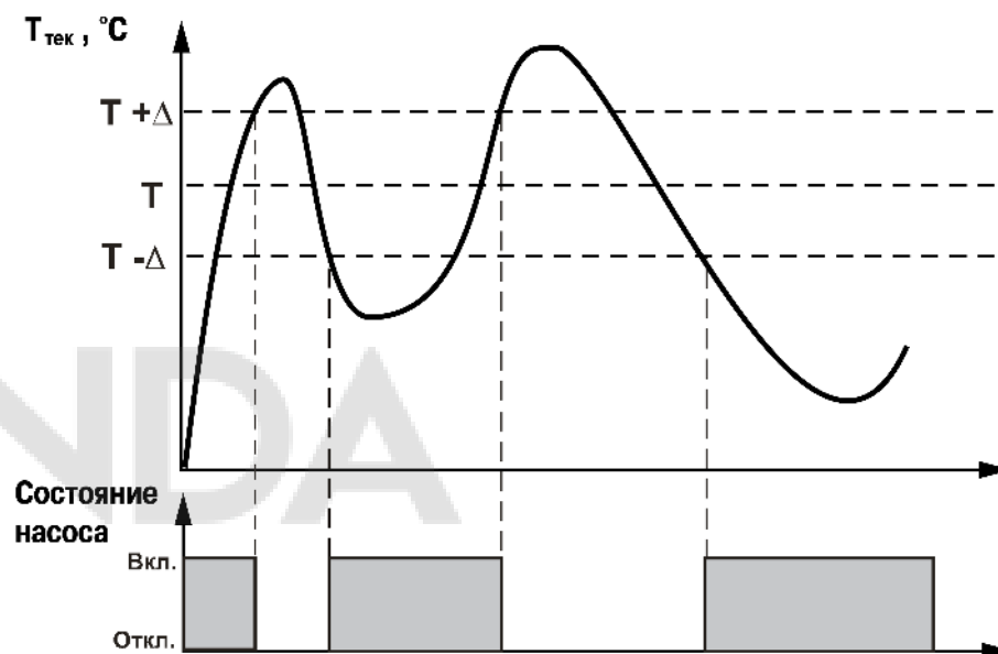
Рисунок 10.1 – Регулирование температуры в зависимости от времени включения насоса
