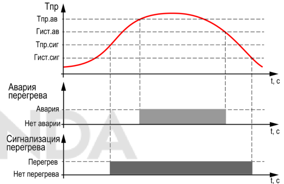
Рисунок 10.10 – Принцип определения и сброса аварии и сигнализации перегрева
