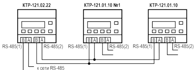
Рисунок 5.2 – Подключение двух KTP-121.03 к KTP-121.02
