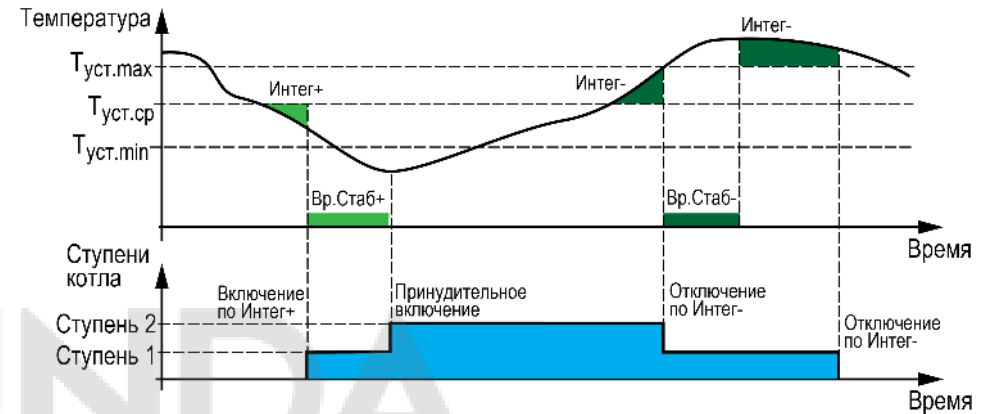
Рисунок 10.2 – Регулирование температуры
