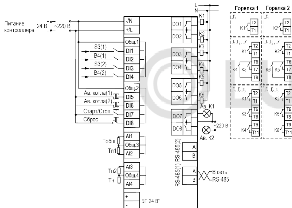
Рисунок 7.4 – Схема подключения КТР–121.02.22 для управления котельной с двумя котлами и контурами ГВС
