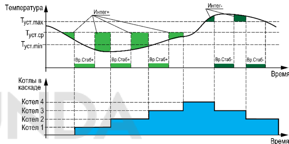
Рисунок 10.6 – Регулирование температуры
