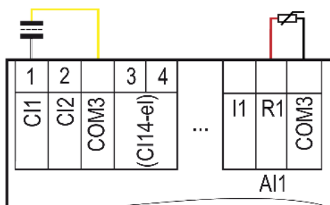
Рисунок 8.7 – Схема подключения кондуктометрического датчика с коррекцией температуры с указанием цвета проводов
