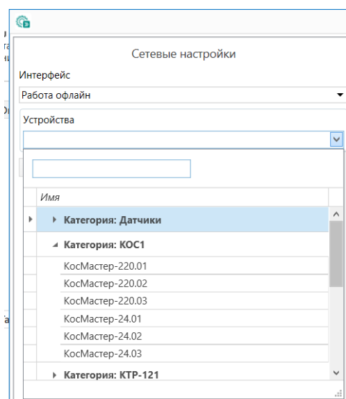
Рисунок 11.4 – Выбор модификации
