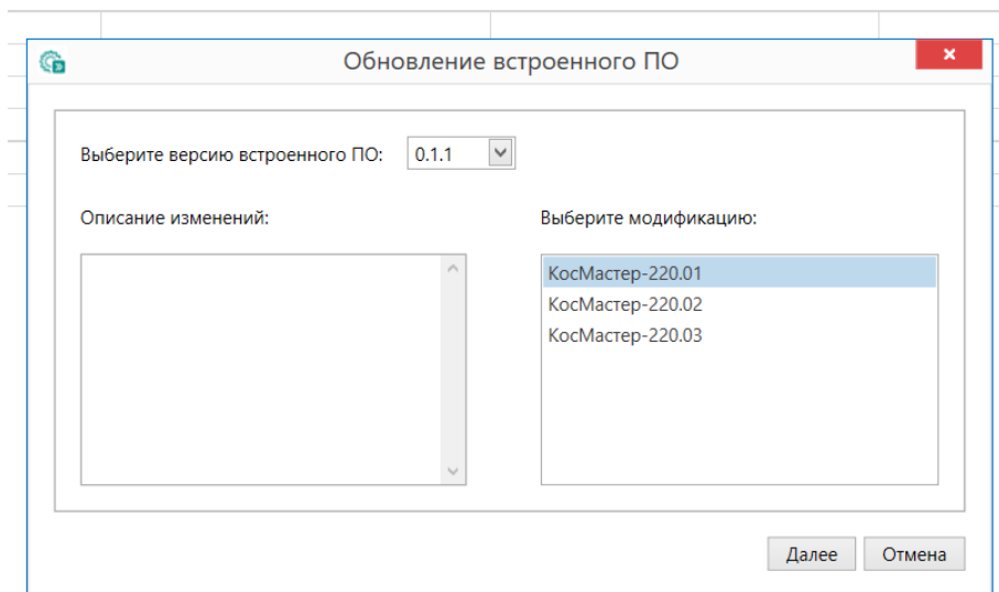
Рисунок 11.7 – Выбор алгоритма
