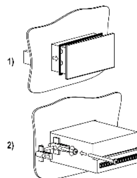
Рисунок 4.1 – Монтаж прибора щитового крепления
