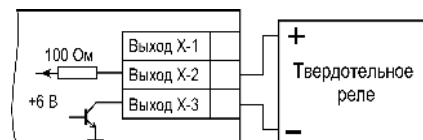
Рисунок 5.6 – Схема подключения к ВУ типа Т
