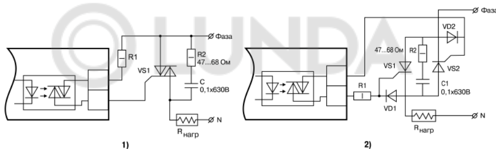
Рисунок 5.5 – Использование симисторной оптопары: 1) для управления силовым симистором, 2) для управления силовыми тиристорами
