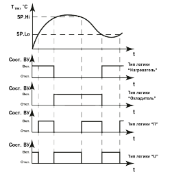
Рисунок 8.1 – Типы логики работы прибора
