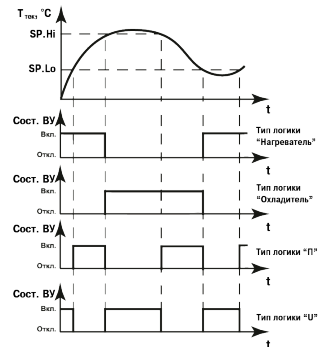
Рисунок 7.1 – Типы логики работы прибора
