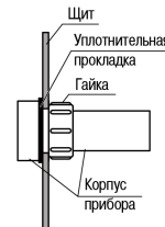
Рисунок 4.1 – Монтаж прибора щитового крепления
