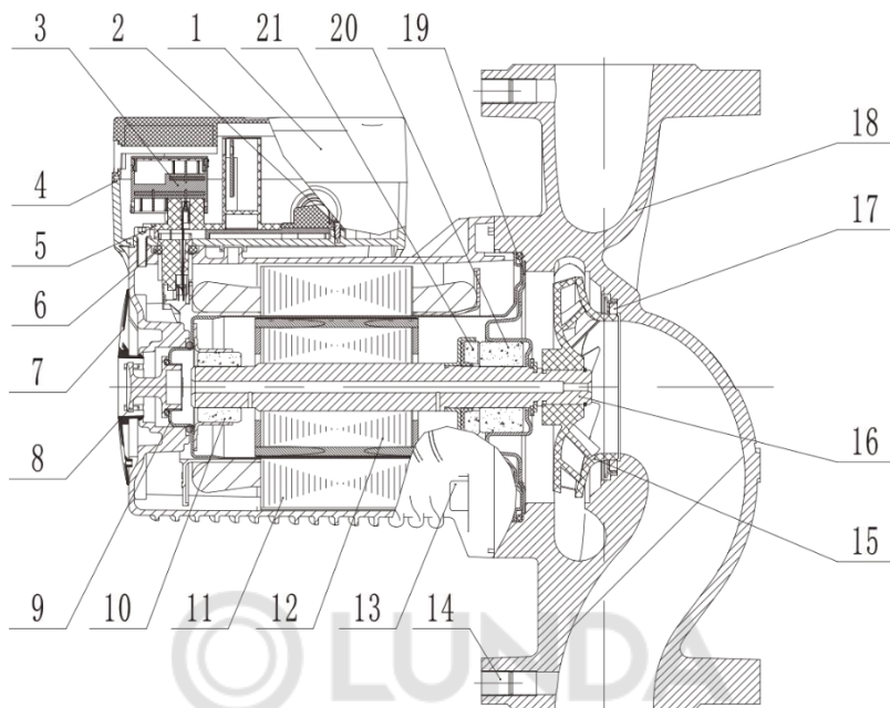
Рис. 2 Вид в разрезе CMS(L)-II
