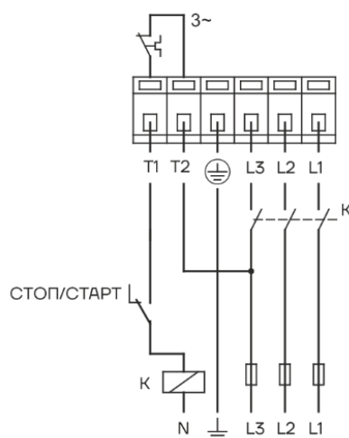
Рис. 14 Схема подключения при использовании внешнего механического пускателя
