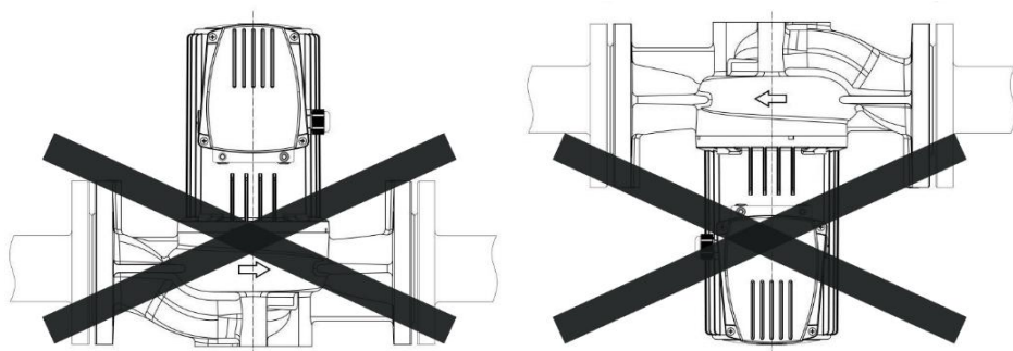
Рис. 6 Недопустимое вертикальное расположение вала насоса
