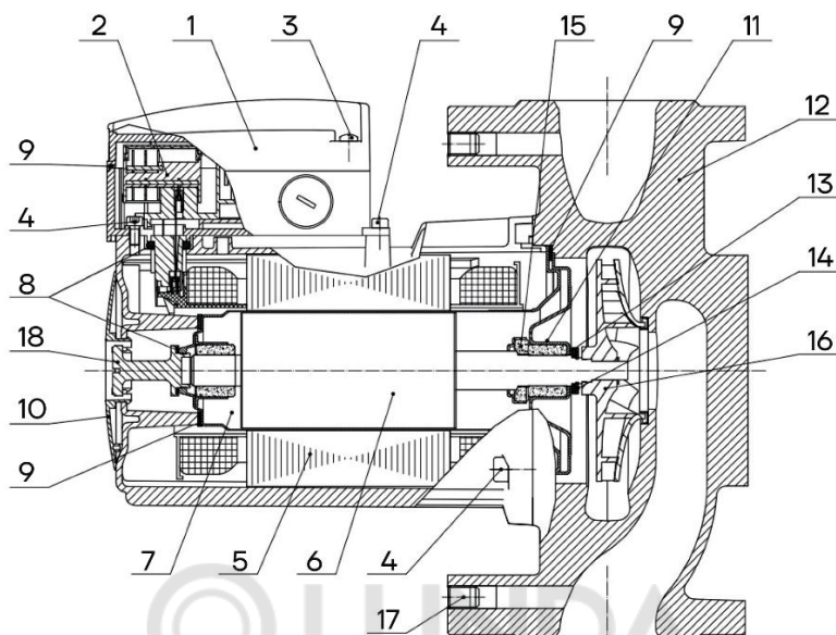
Рис. 1 Вид в разрезе CMS(L)-I
