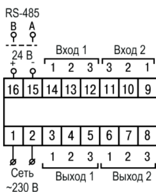
Рисунок 5.5 – Общая схема подключения 2TRM1–Щ5
