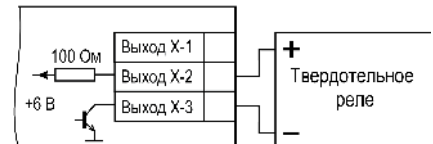
Рисунок 5.19 – Схема подключения нагрузки к ВУ типа «Т»
