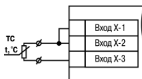
Рисунок 5.11 – Двухпроводная схема подключения ТС
