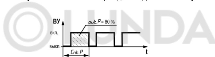
Рисунок 7.6 – Мощность дискретного ВУ
