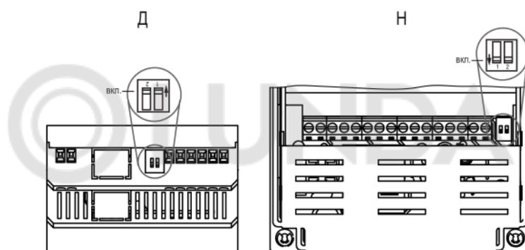
Рисунок 5.16 – Расположение DIP-переключателей для корпусов Д и Н
