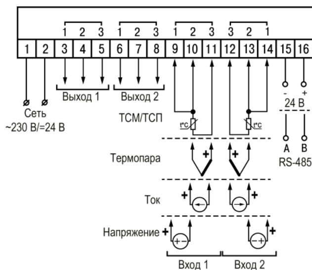
Рисунок 5.4 – Общая схема подключения 2TRM1–Щ1/Щ2
