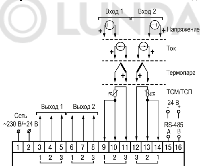
Рисунок 5.6 – Общая схема подключения 2TRM1–Д
