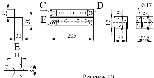
Габаритные и крепежные размеры
