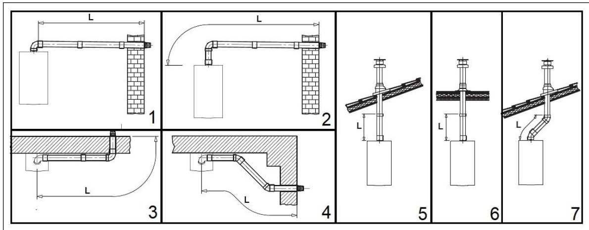
Рис. 5. Монтаж коаксиальной трубы
