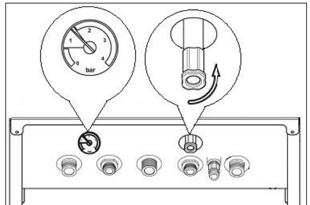
Рис.7 Кран подпитки и манометр
