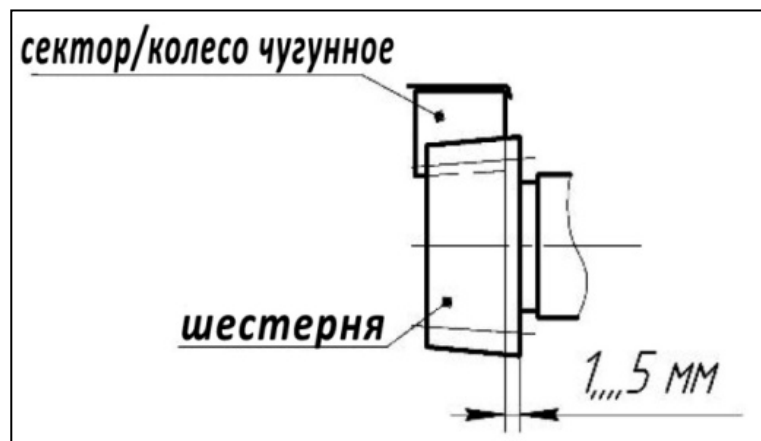
Рис. 10. Допустимый зазор
