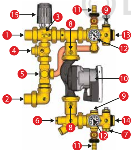
Составные элементы узла R557RY042
