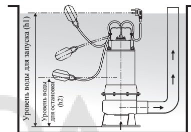
Схема запуска и отключения насоса в зависимости от уровня воды
