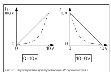
Рис. 5: Характеристики при перестановке DIP-переключателя 7
