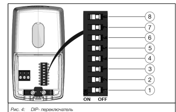
Рис. 4: DIP-переключатель
