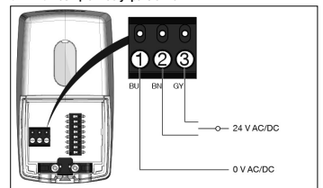
Рис. 7: Подключение для 3-позиционного управления
