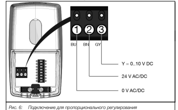
Рис. 6: Подключение для пропорционального регулирования
