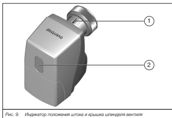
Рис. 9: Индикатор положения штока и крышка шпинделя вентиля
