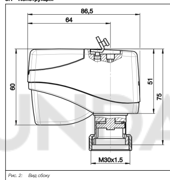
Рис. 2: Вид сбоку
