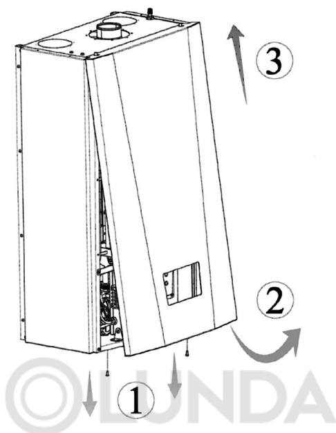
Рис. 10. Снятие лицевой крышки
