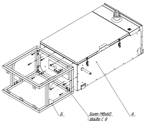
Рис. 6. Сборка постамент с котлом
