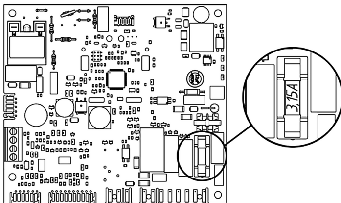
Рис. 13. Расположение предохранителя
