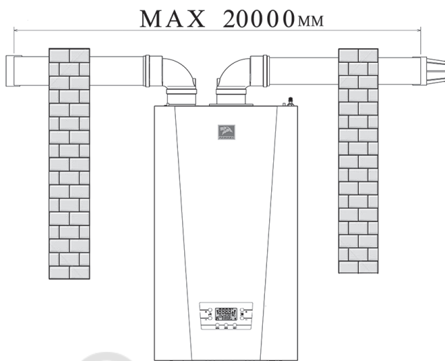
Рис. 5. Раздельный дымоход
