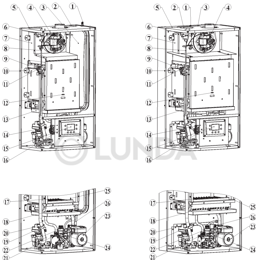
Рис.1. Конструкция котла:
