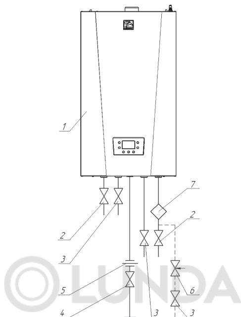
Рис.3. Требования к подключению котла
