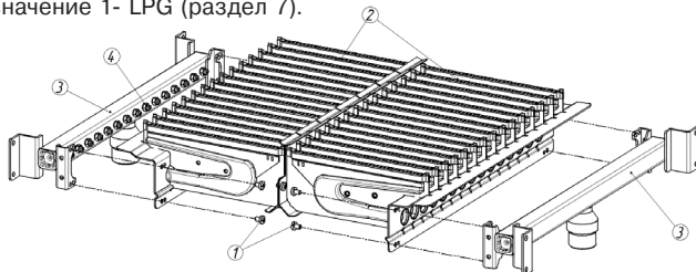
Рис. 9. Замена сопел
